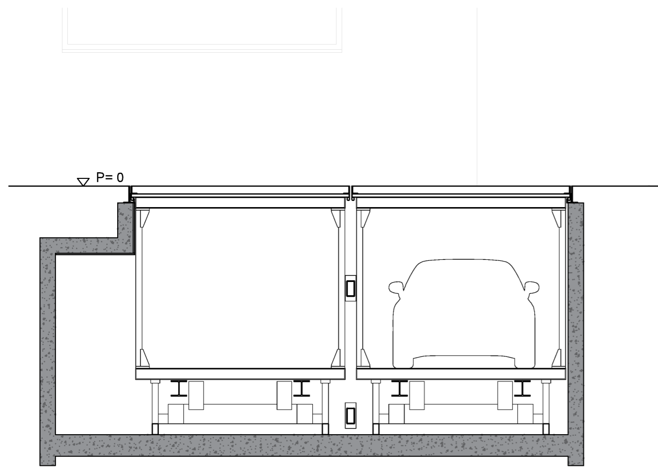
Doorsnede A (Positie omlaag) 1:50
