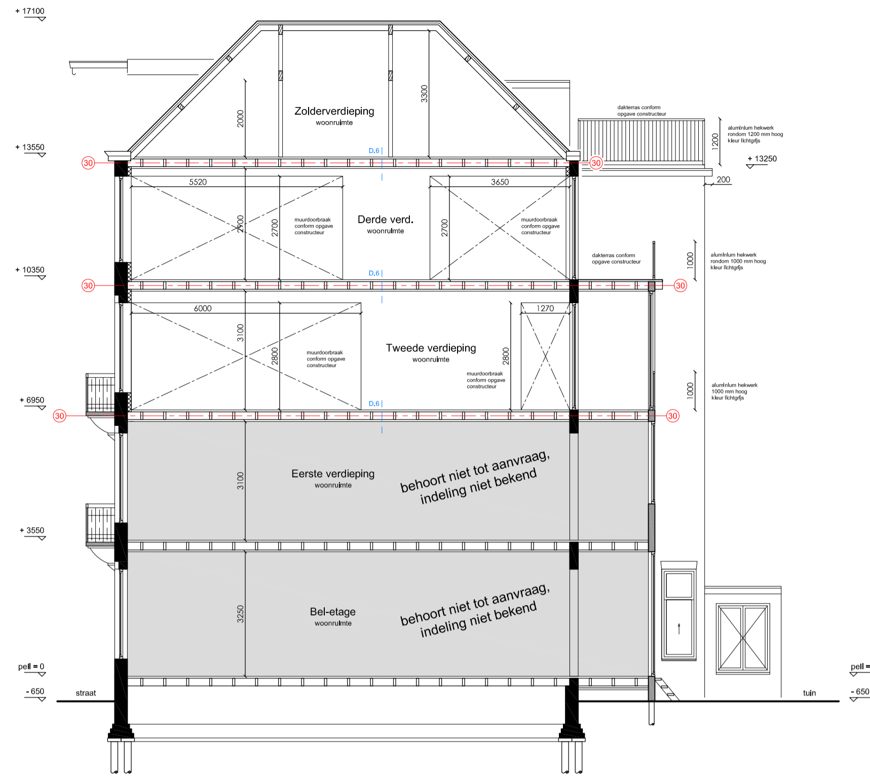
Doorsnede A-A
