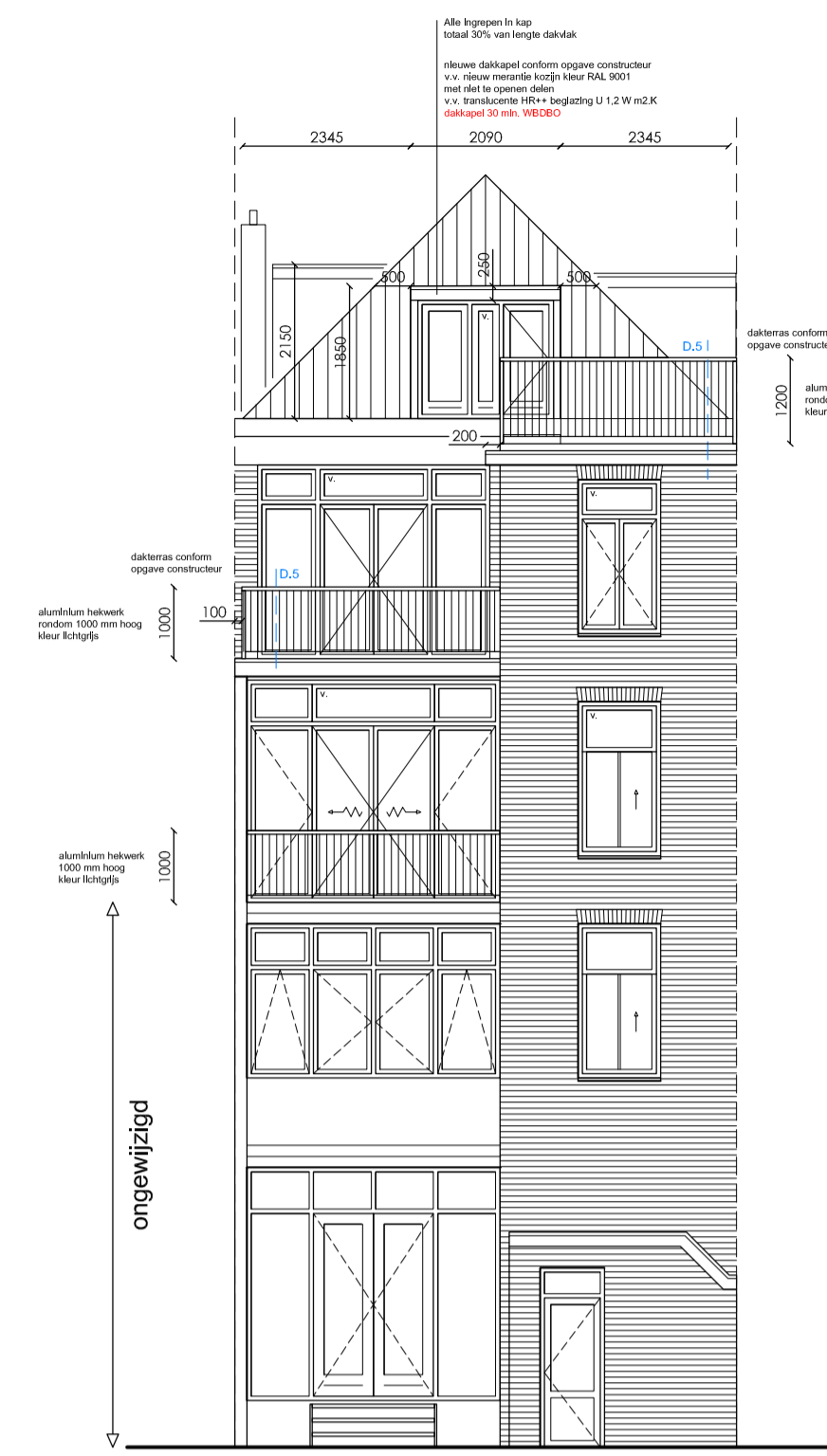
Achtergevel
