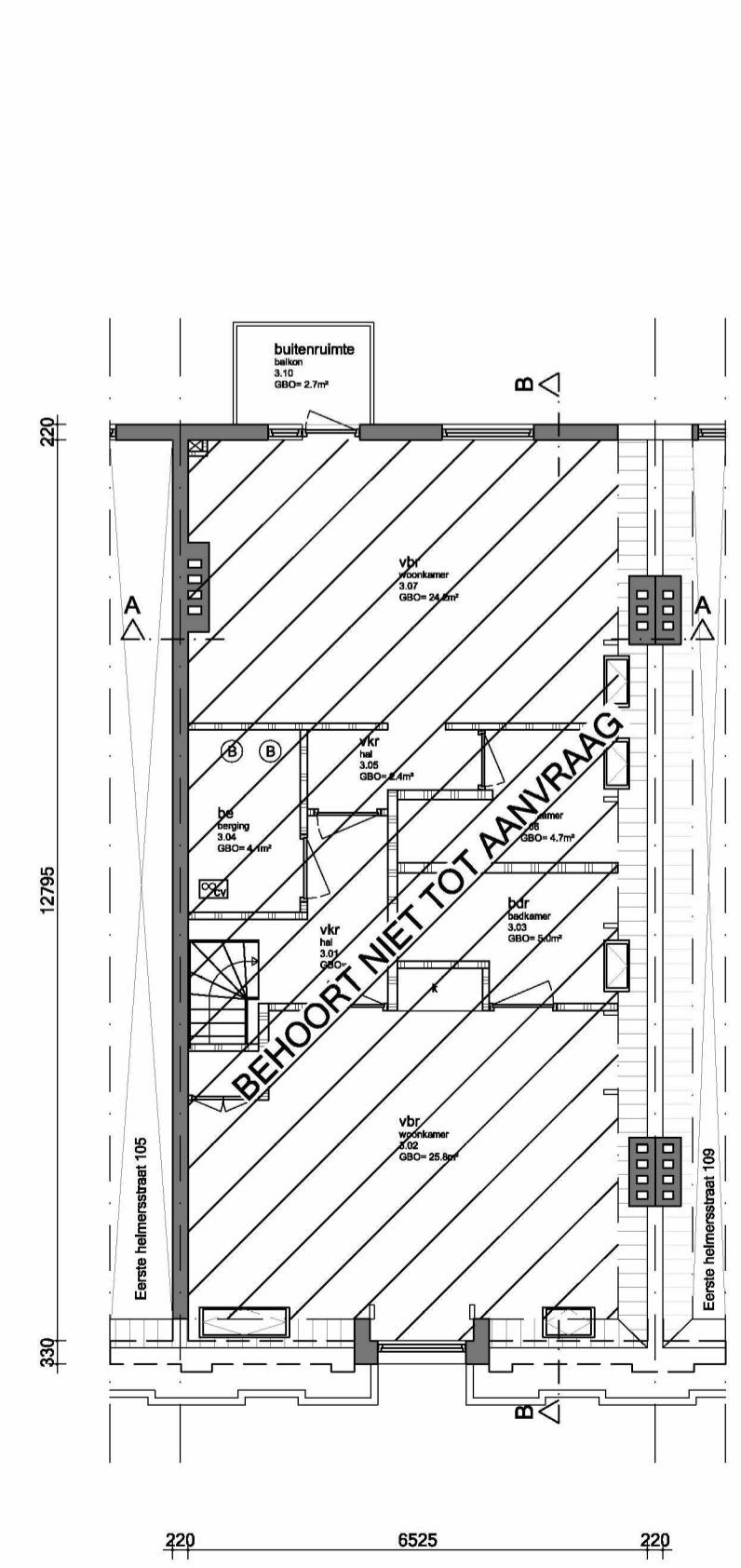
Derde verdieping
