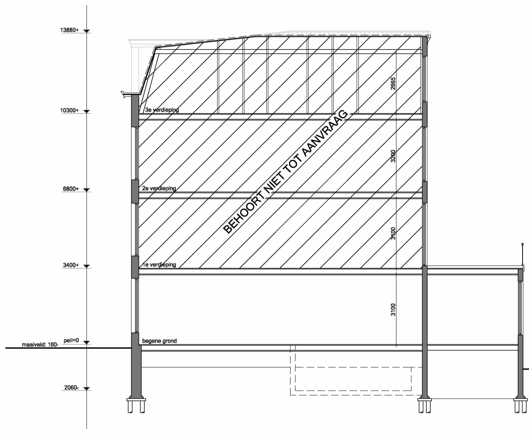
Doorsnede B-B
