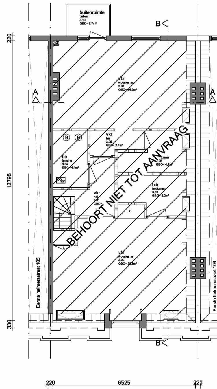
Derde verdieping
