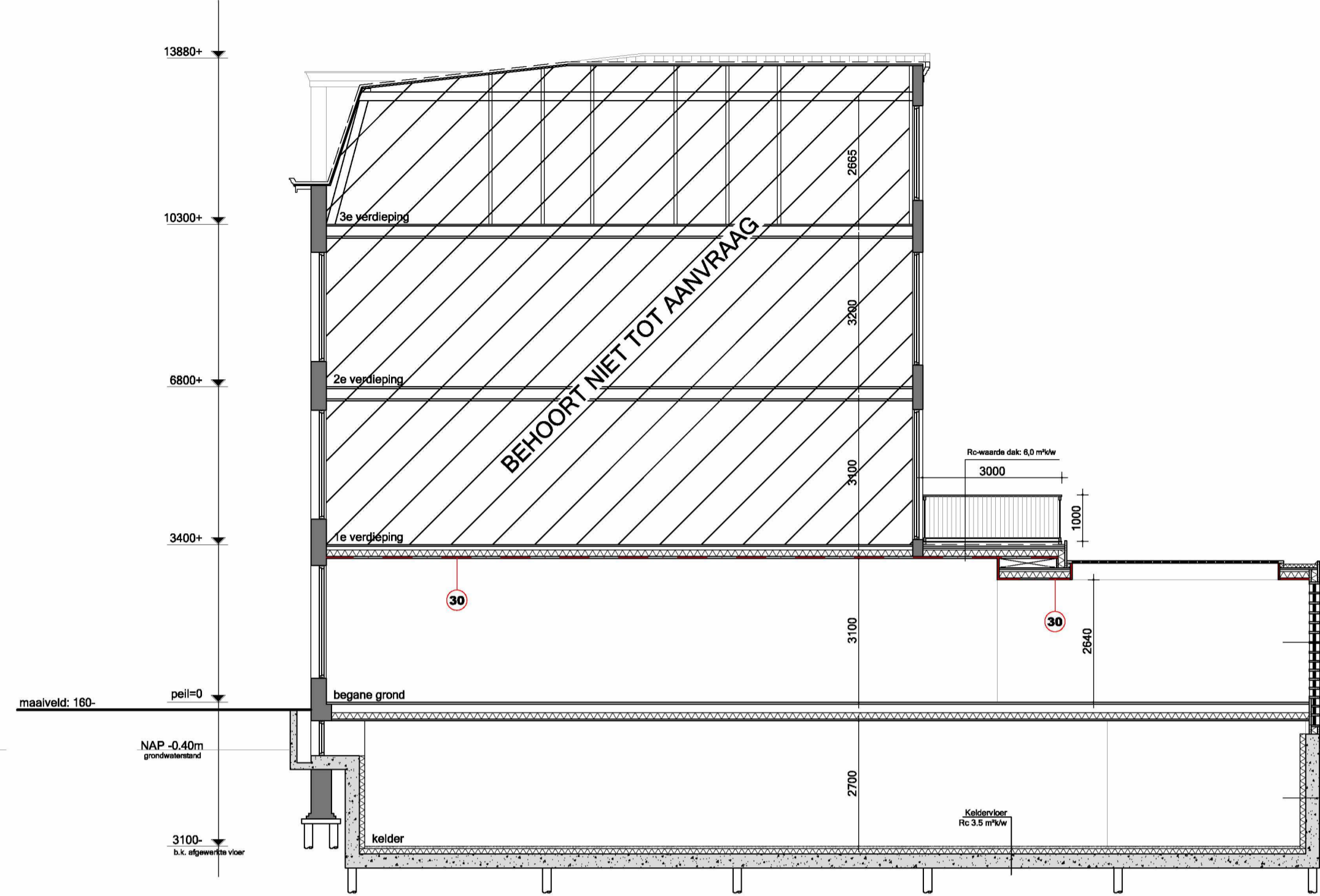
Doorsnede B-B
