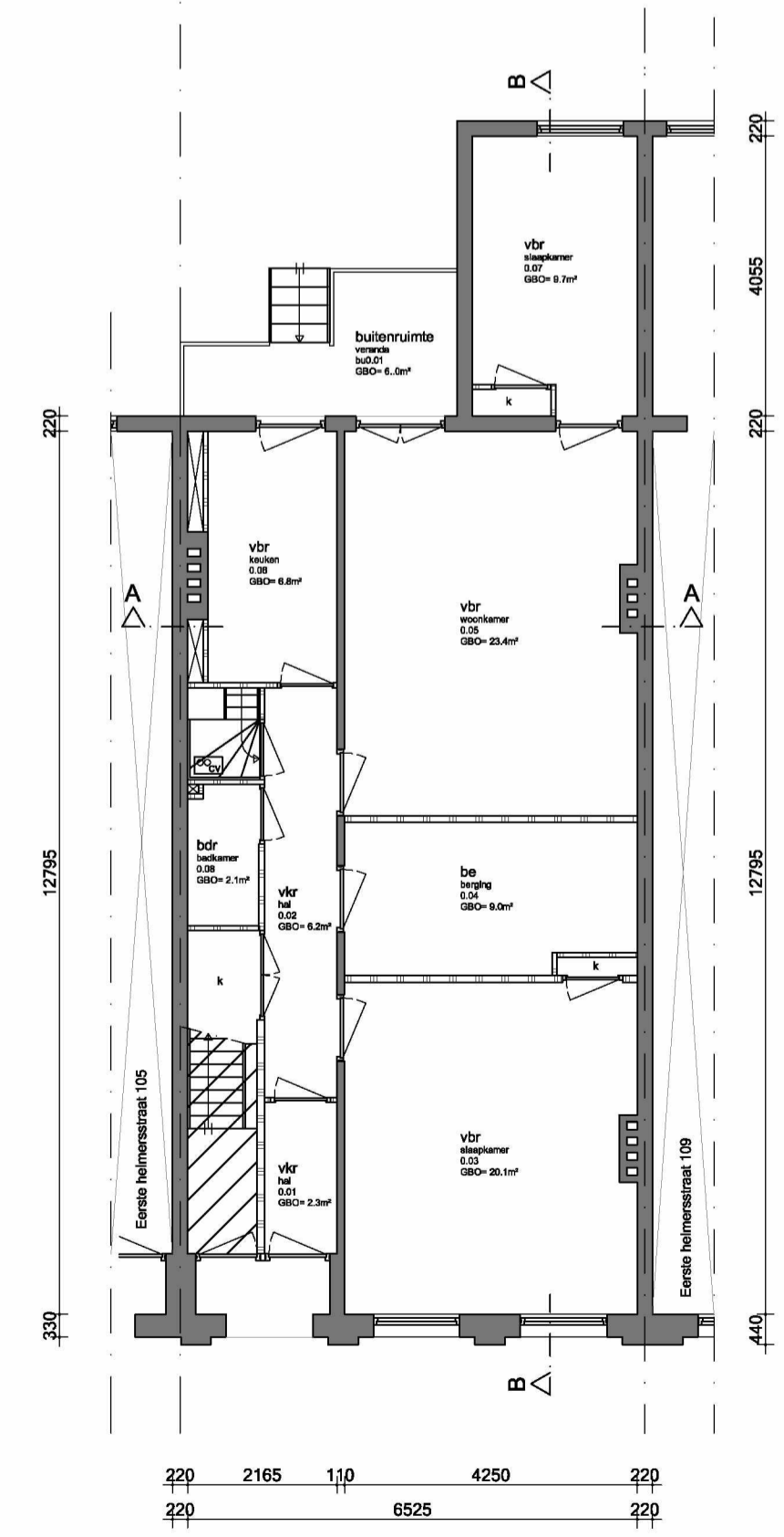
Begane grond
