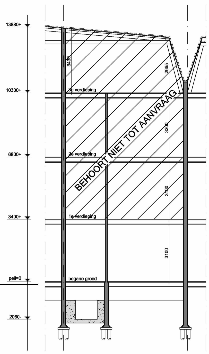
Doorsnede A-A
