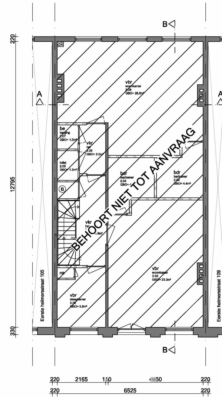
Tweede verdieping
