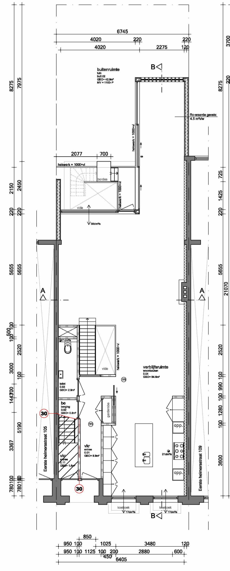
Begane grond
