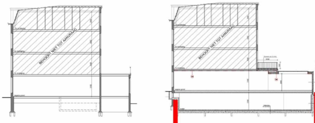
Figuur 1 – situatie project (links bestaand, rechts nieuw, damwanden = rood)
