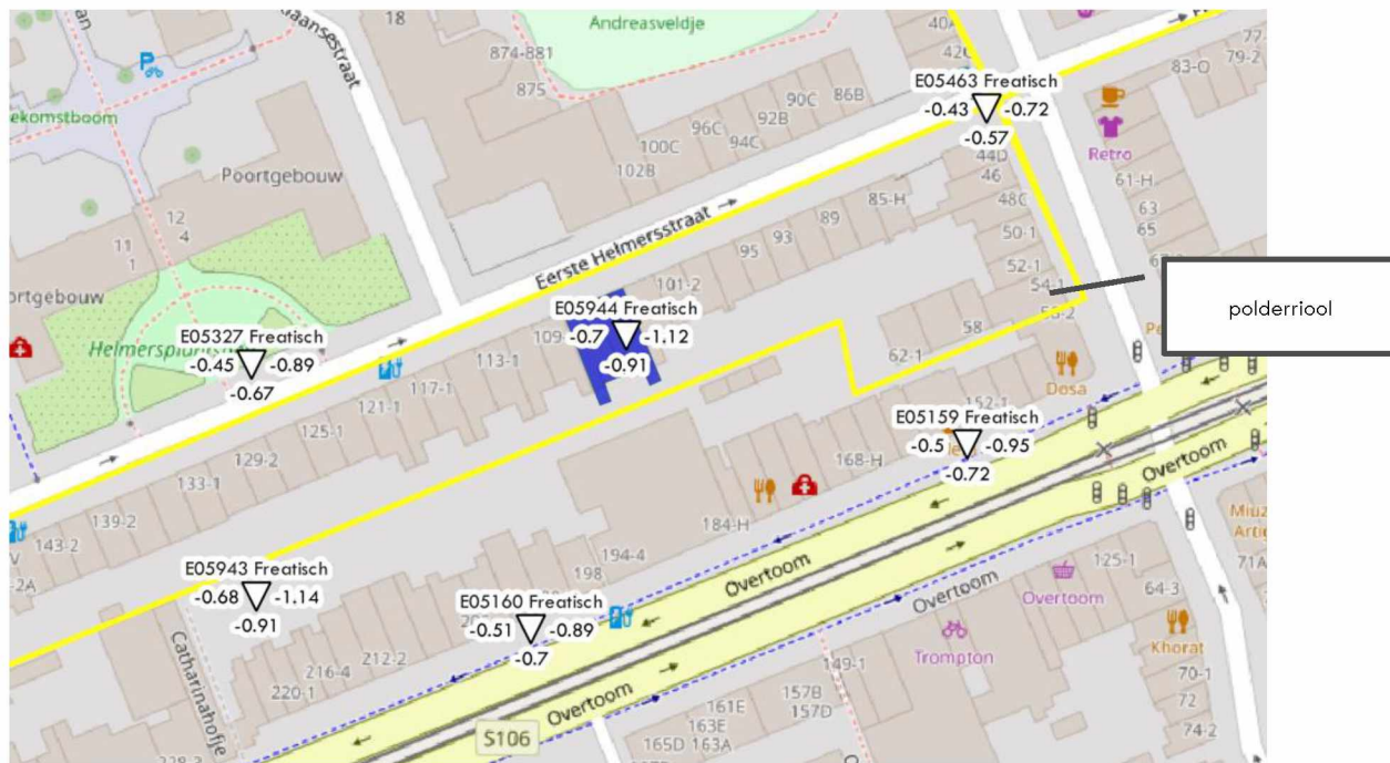
Figuur 6 – grondwaterstanden ten opzichte van NAP [m] (boven driehoek=peilbuis naam, onder driehoek=gemiddelde grondwaterstand, links driehoek=maatgevend hoge grondwaterstand, rechts driehoek=maatgevende lage grondwaterstand)
