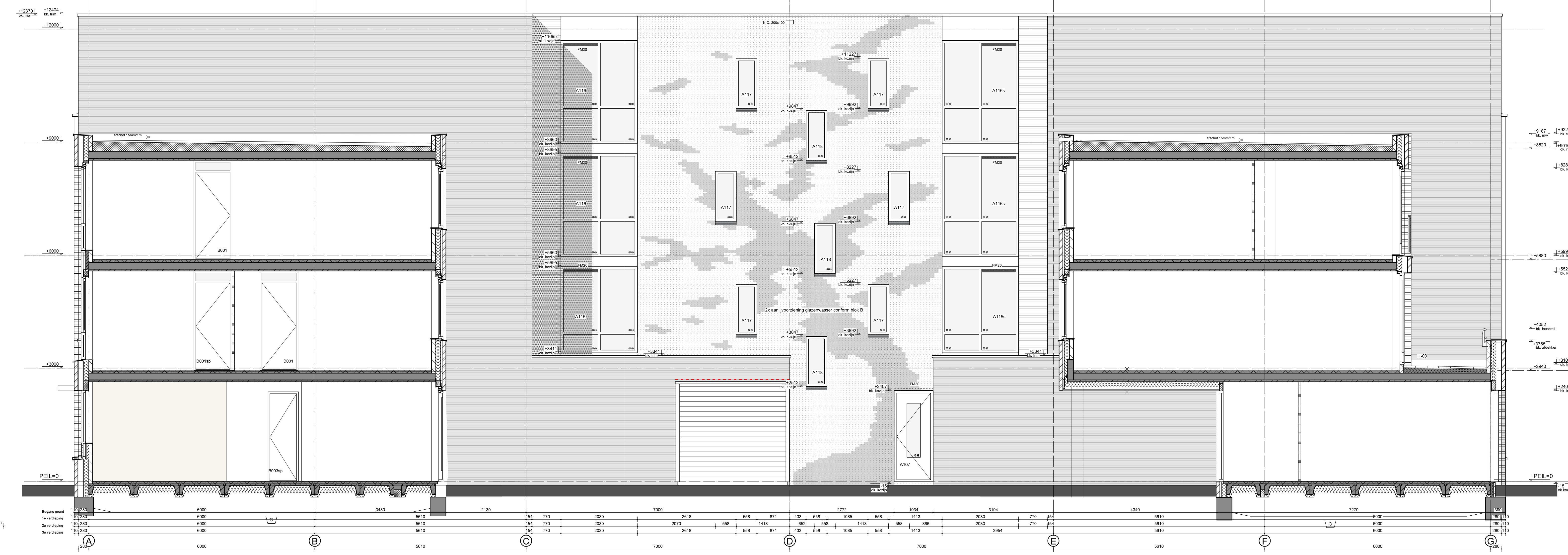
ACHTERGEVEL
