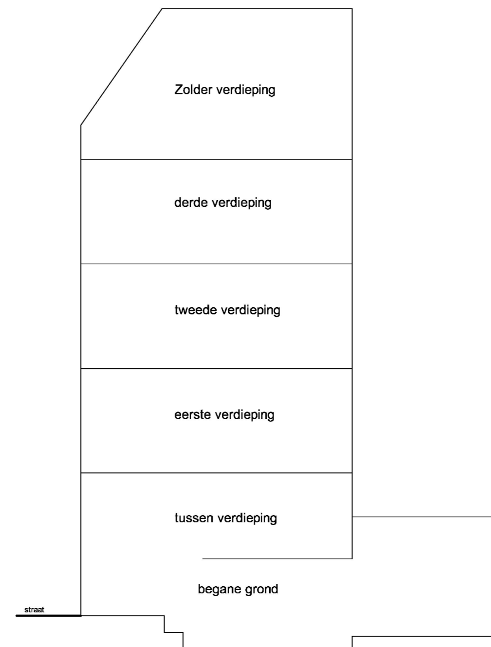
Doorsnede schaal 1:100
