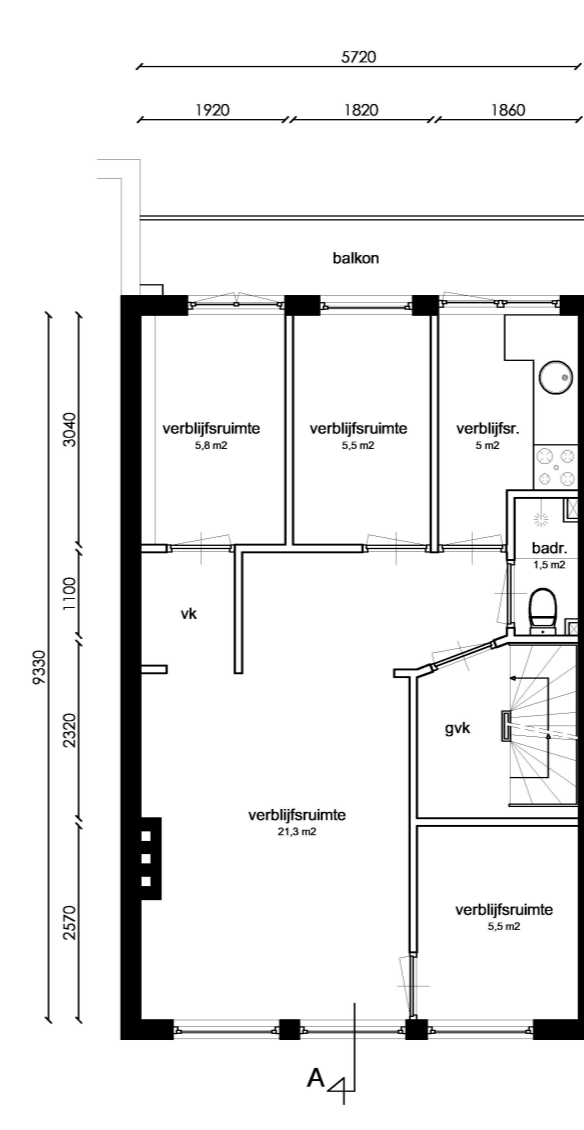
Tweede verdieping
