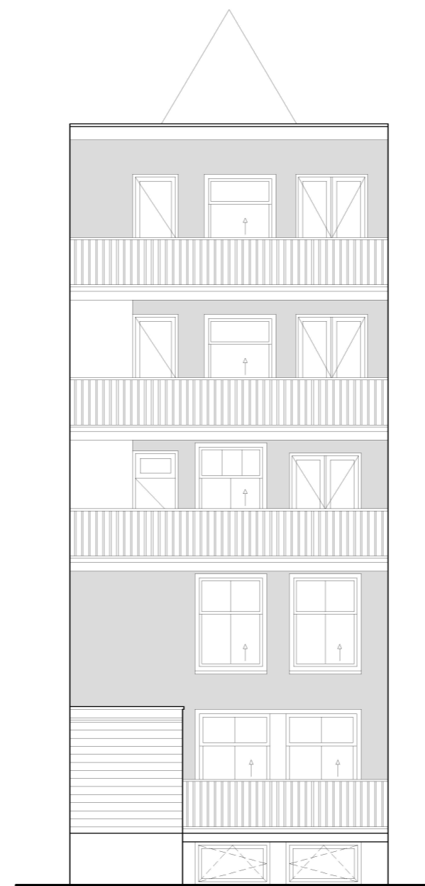
Achtergevel
