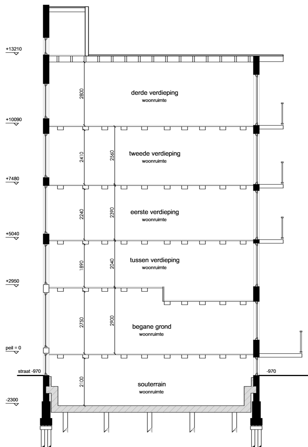
Doorsnede A-A
