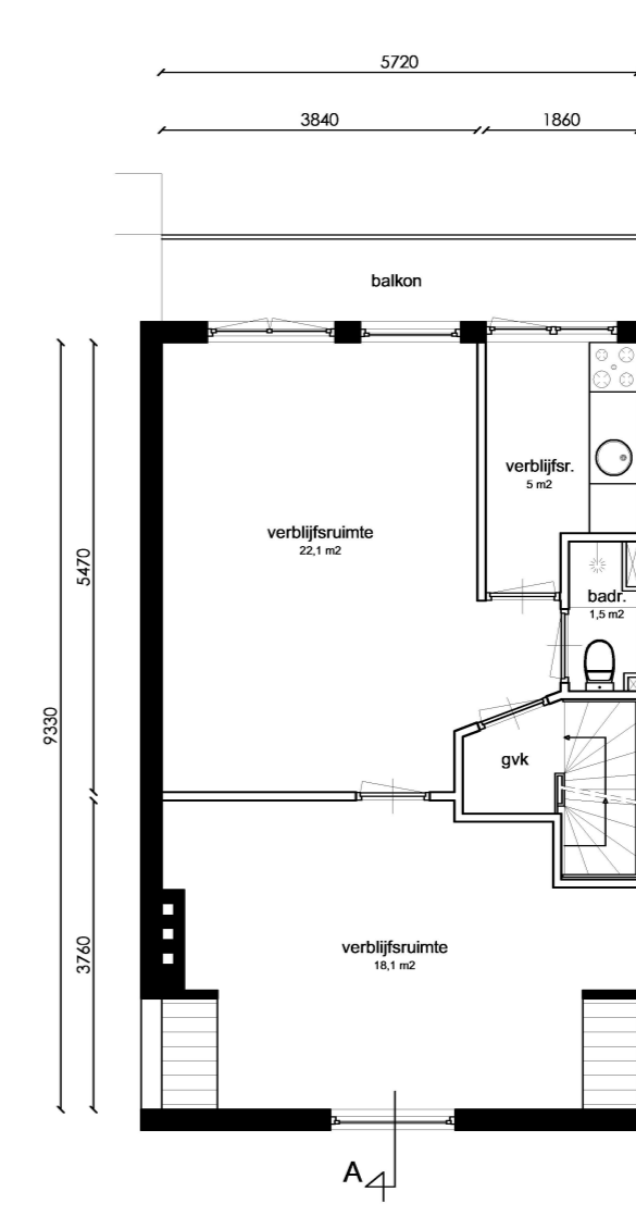
Derde verdieping
