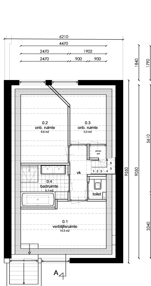
Souterrain
