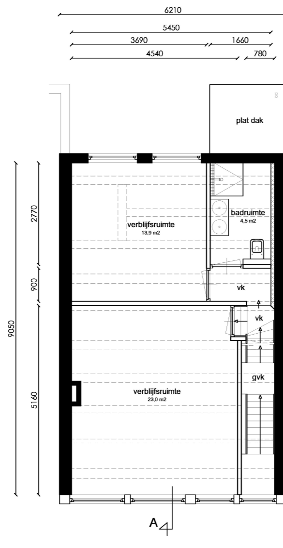
Tussen verdieping
