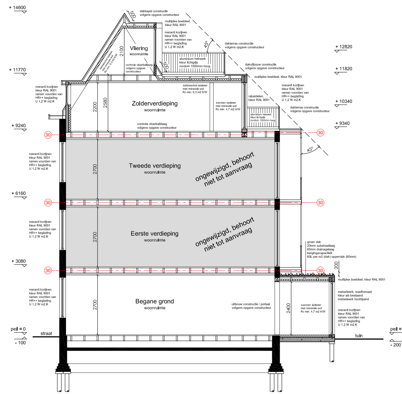
Doorsnede A-A
