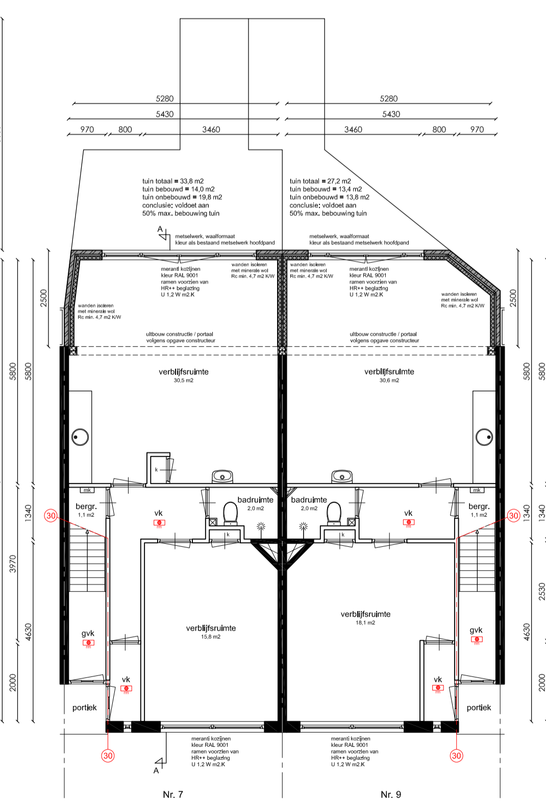
Begane grond
