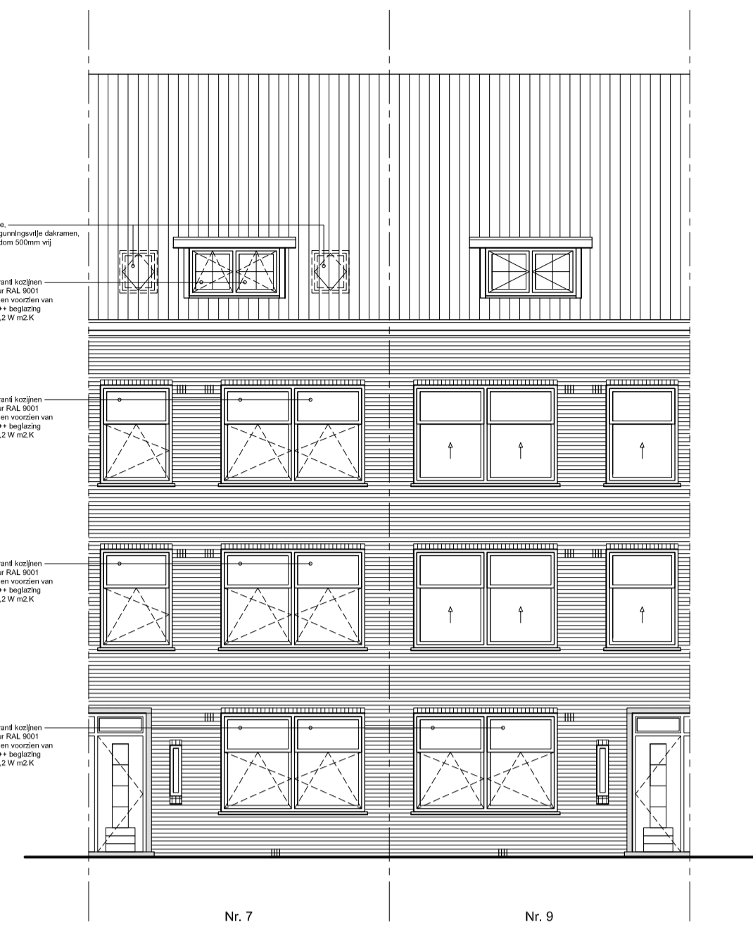
Voorgevel
