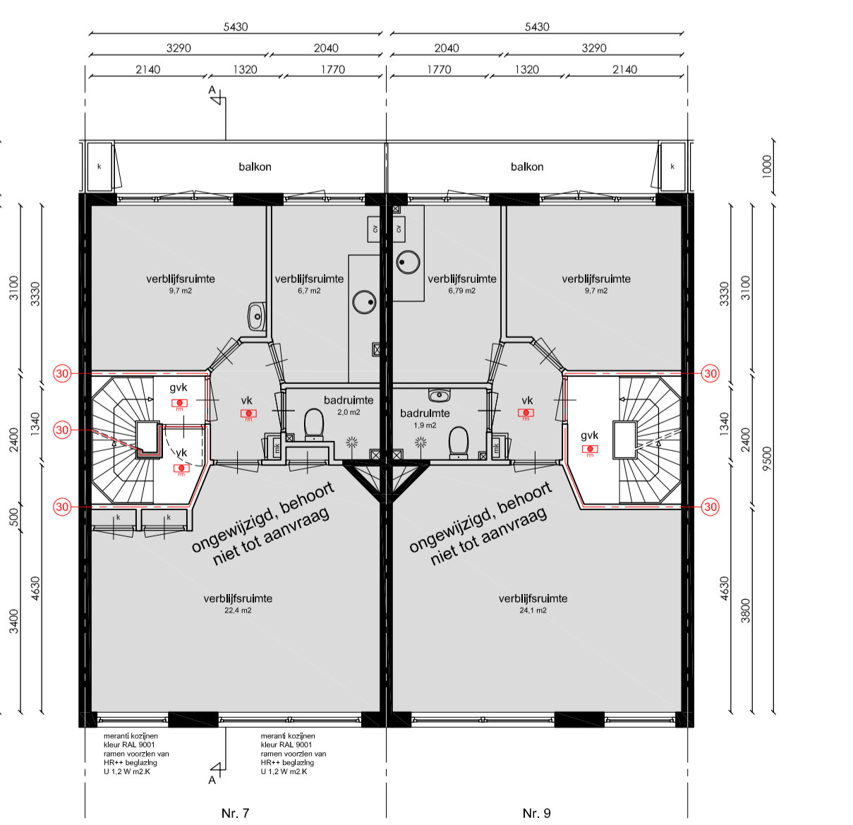
Tweede verdieping
