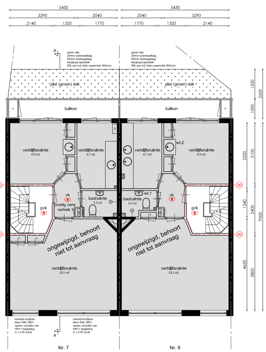
Eerste verdieping
