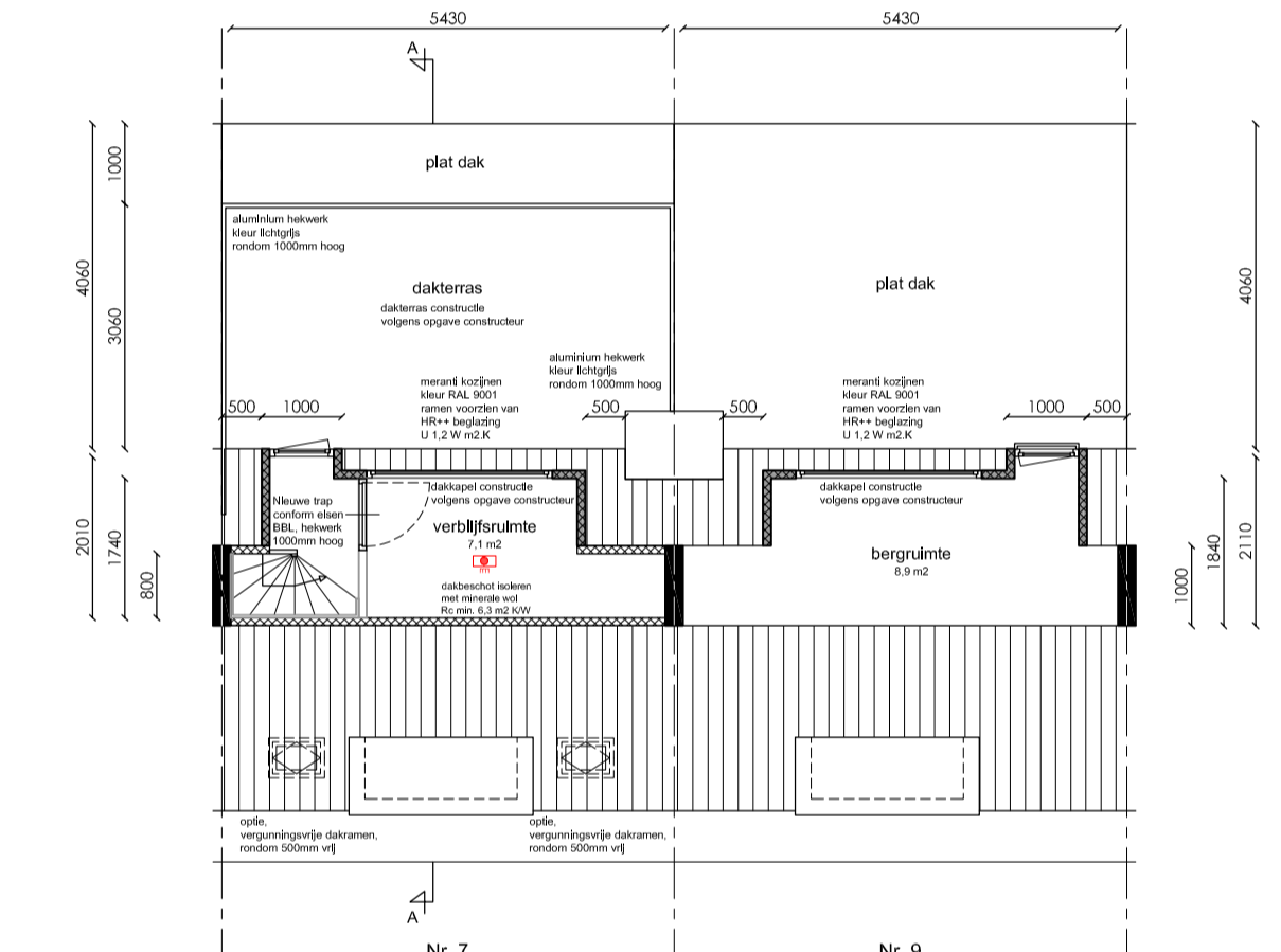
Vliering
