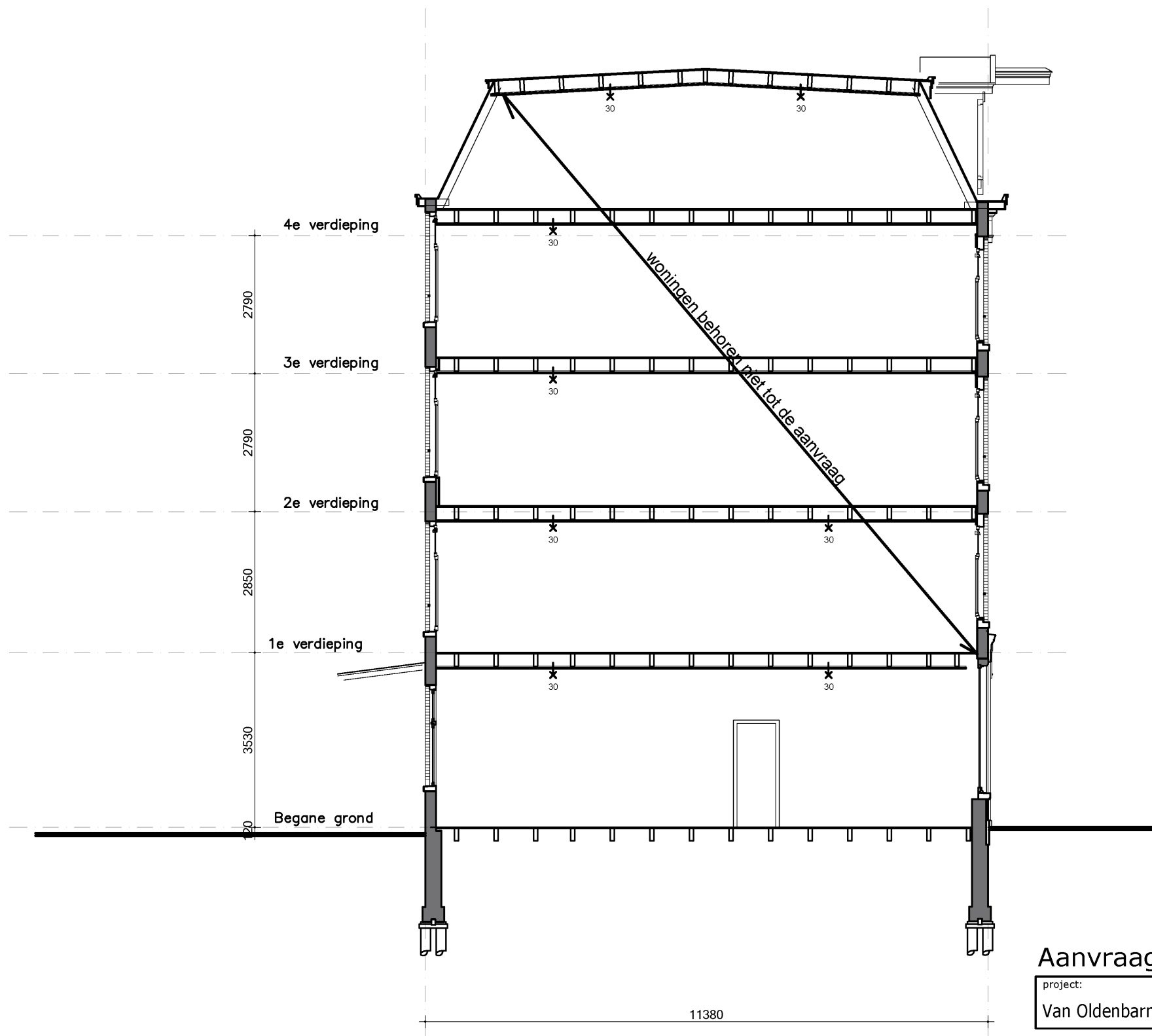
Doorsnede B-B
