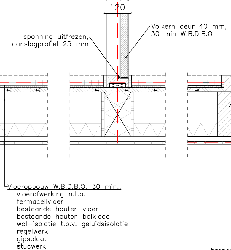
Detail P2 onderaansluiting niet dragende woningscheidende wand
