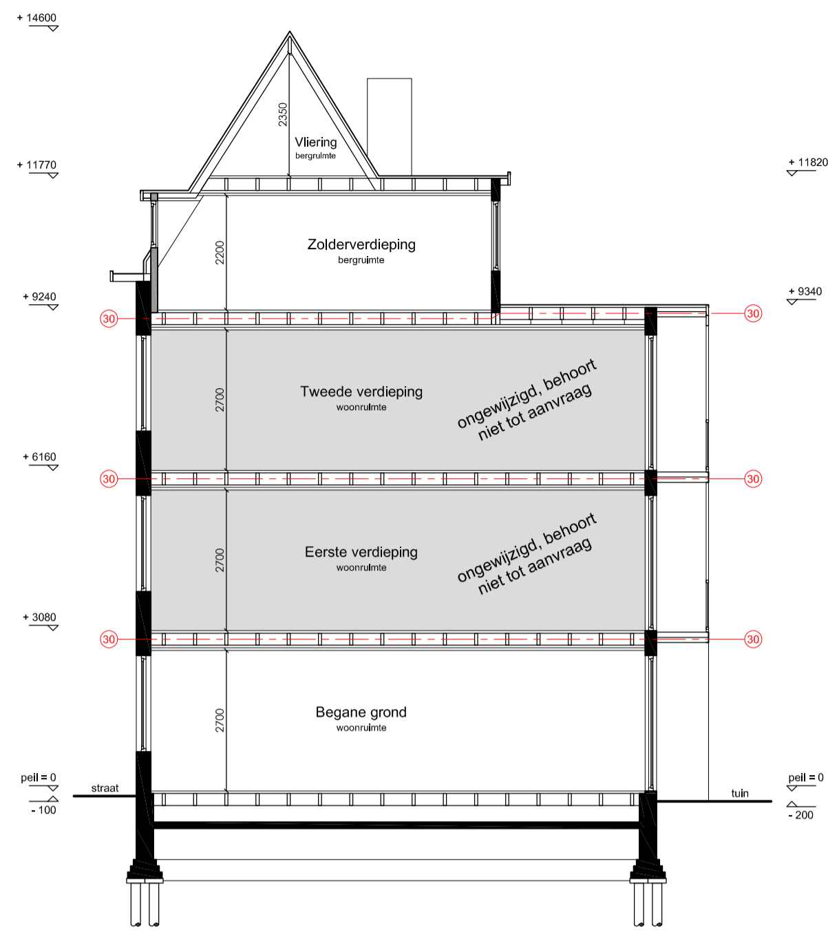
Doorsnede A-A
