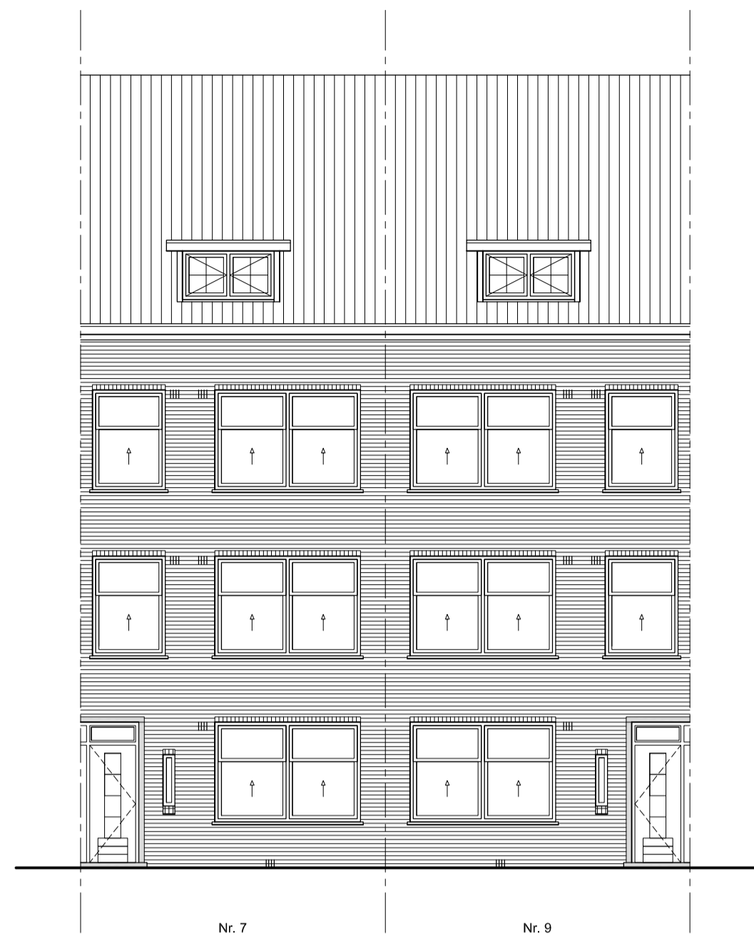
Voorgevel
