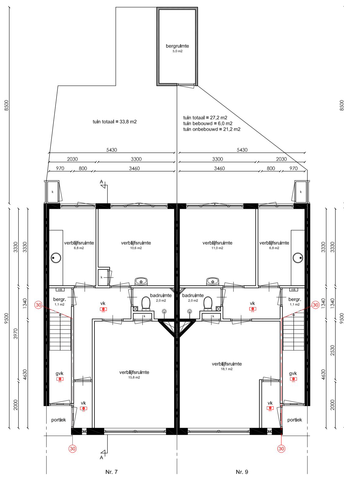
Begane grond
