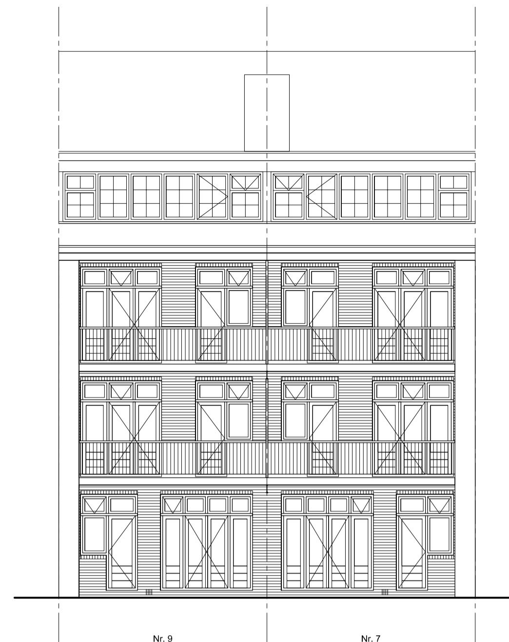
Achtergevel
