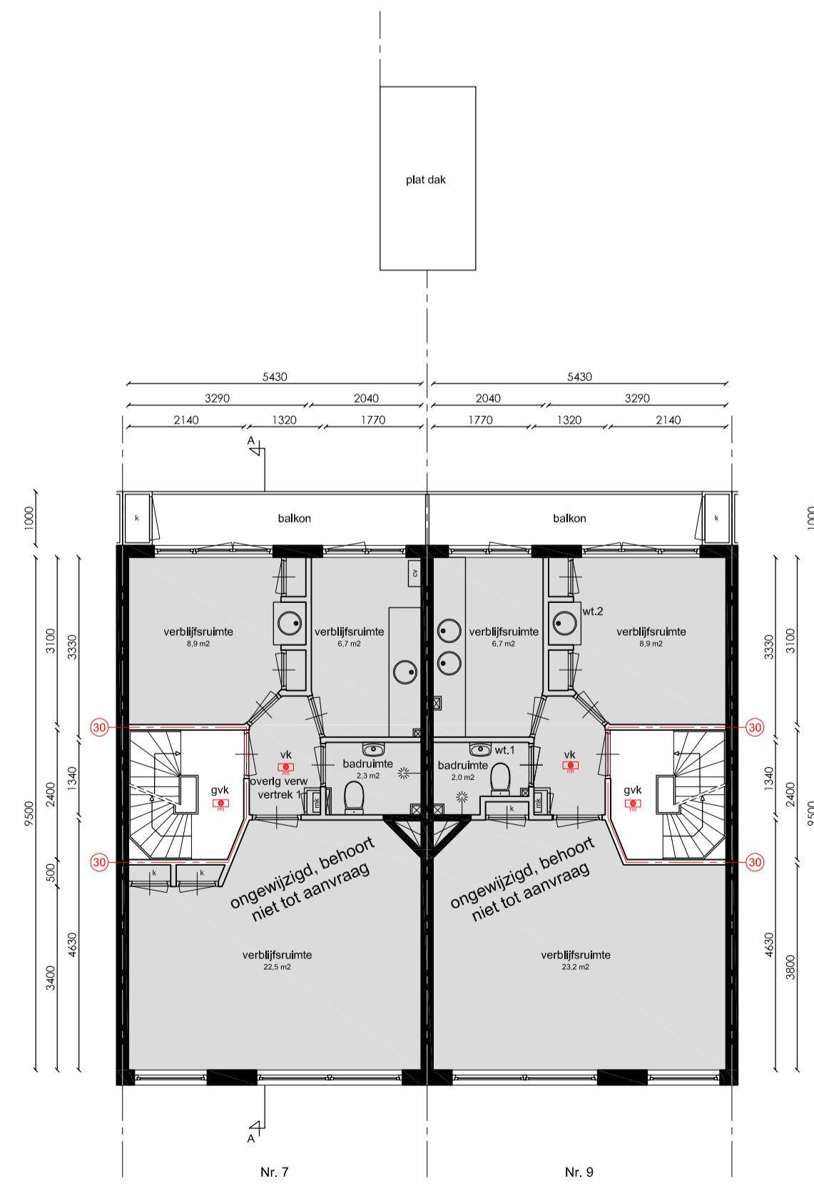
Eerste verdieping
