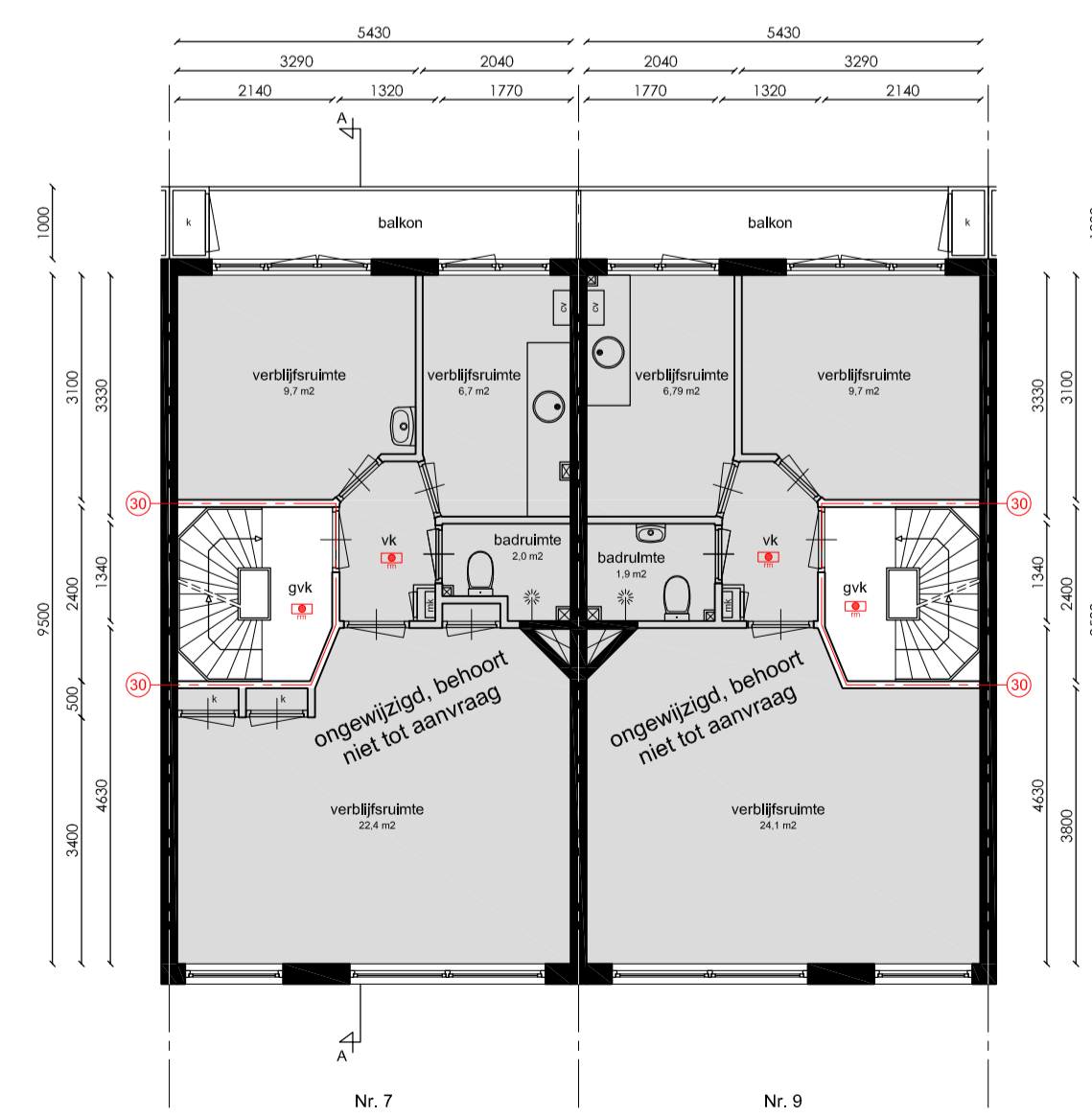
Tweede verdieping
