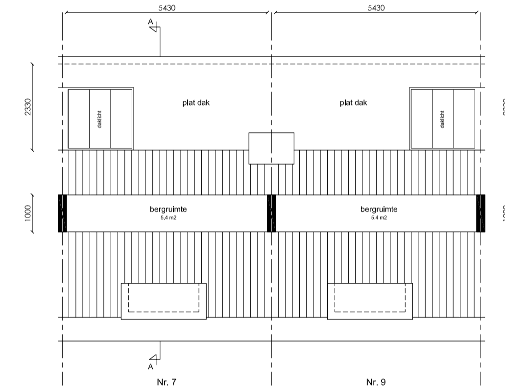
Vliering
