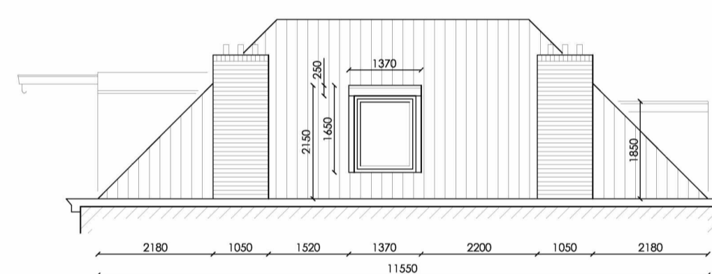
Rechter zijgevel
