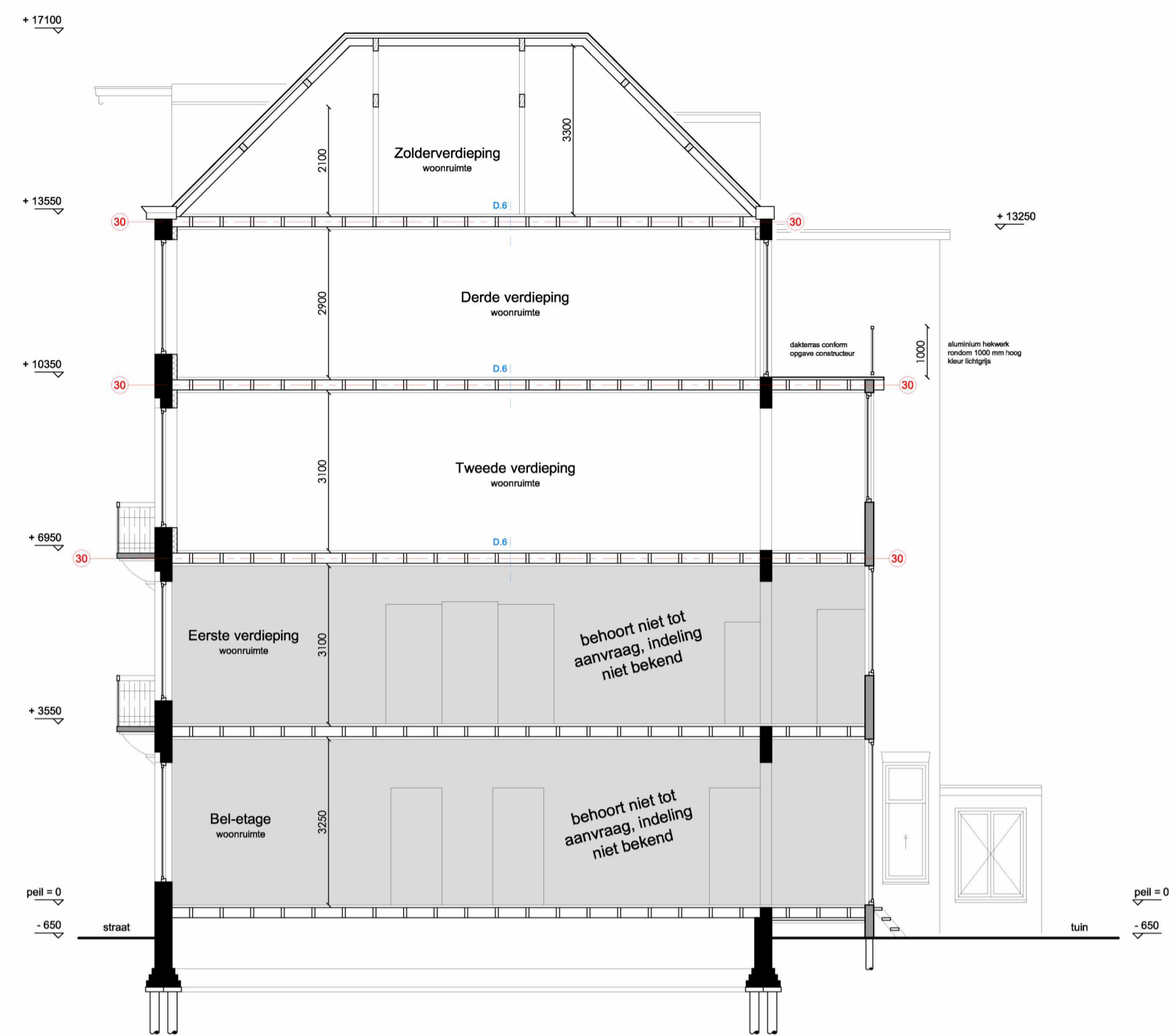
Doorsnede A-A
