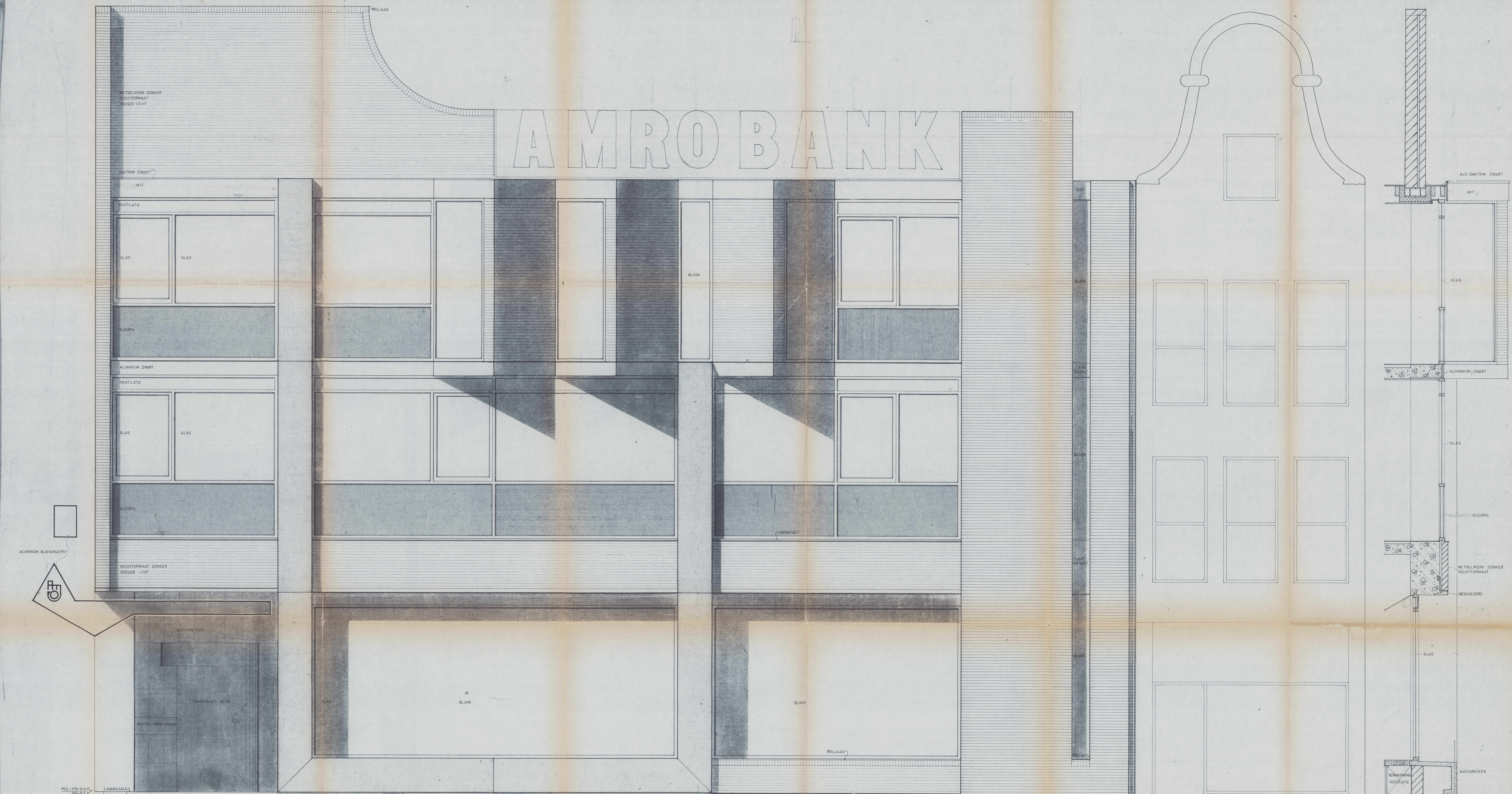
GEVEL HAARLEMMERDIJK
