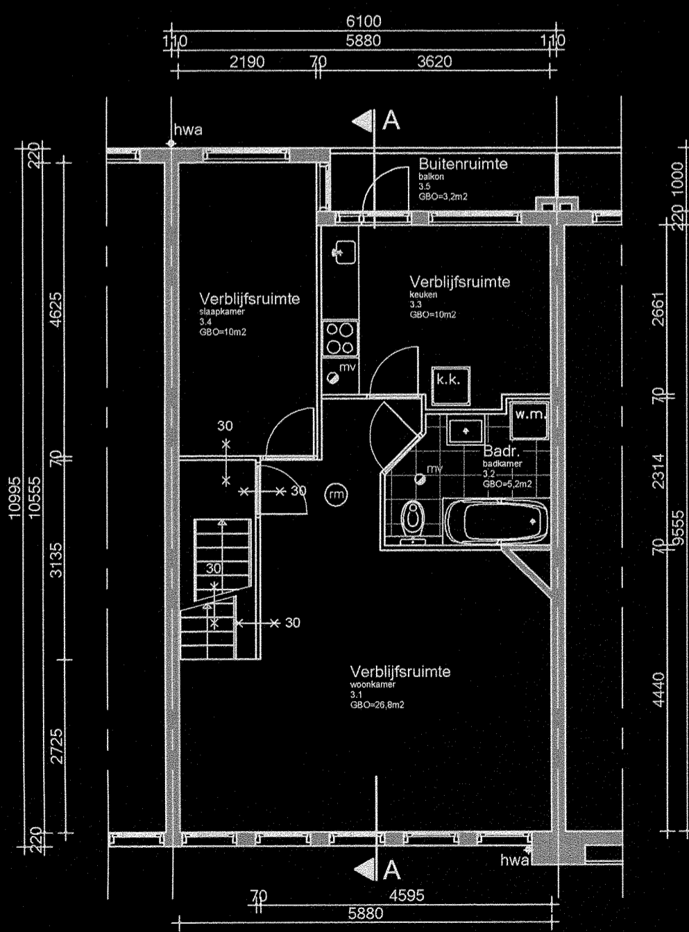
3e verdieping
