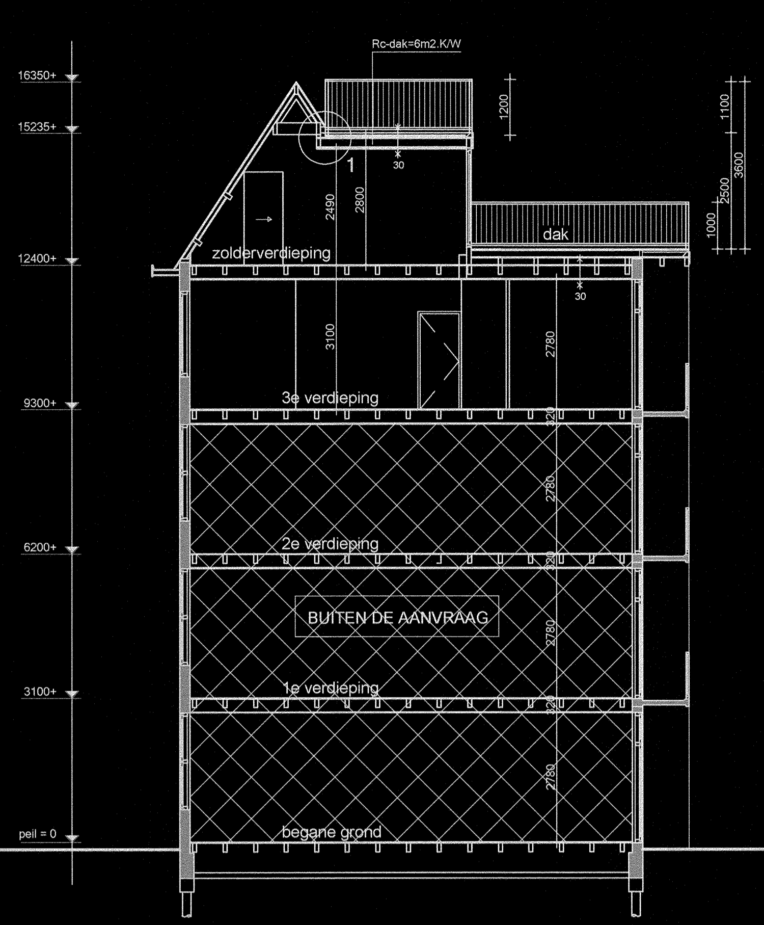
doorsnede A-A
