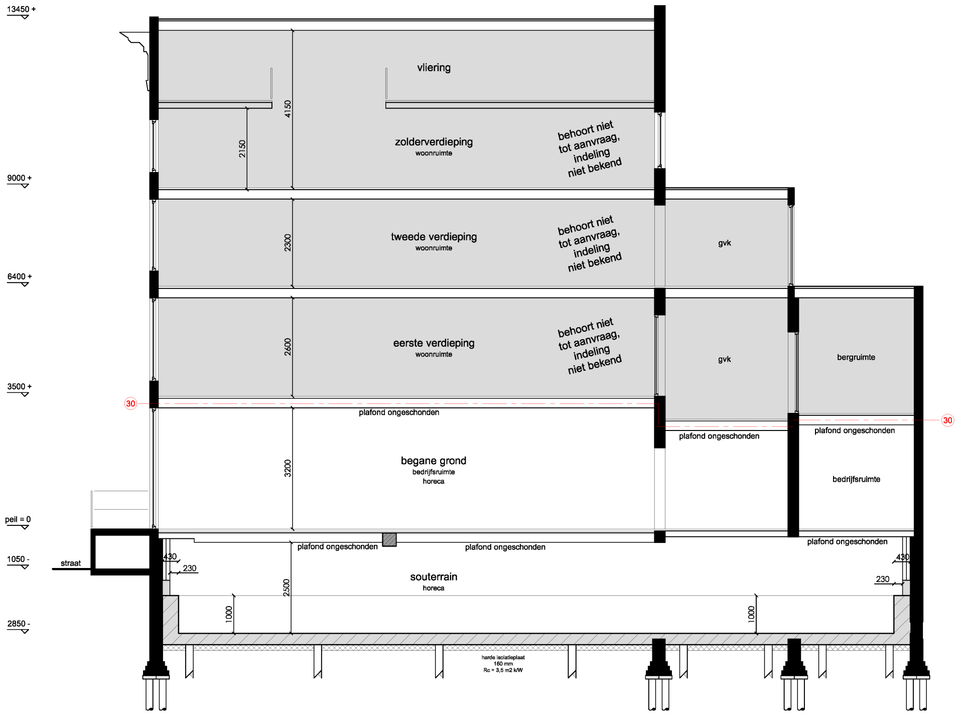
Doorsnede A-A
