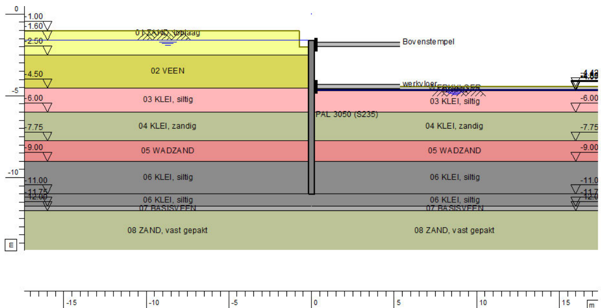
figuur 5: bouwfase 3, maximale ontgraving met afstempeling vloer op damwand
