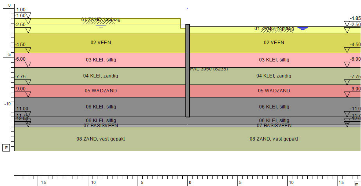
figuur 3: Bouwfase 1, ontgraving tot ca. NAP -1,85 m
