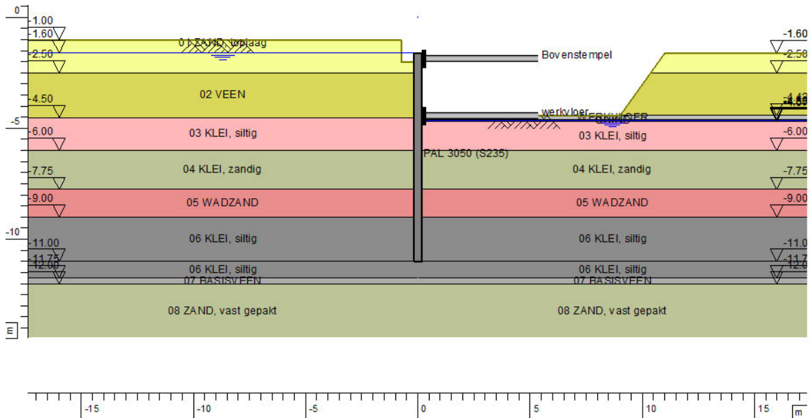
figuur 4: Bouwfase 2, strookgewijs ontgraven tot ca. NAP -4,875 m met daarop 0,3 m zand en 0,15 m werkvloer
