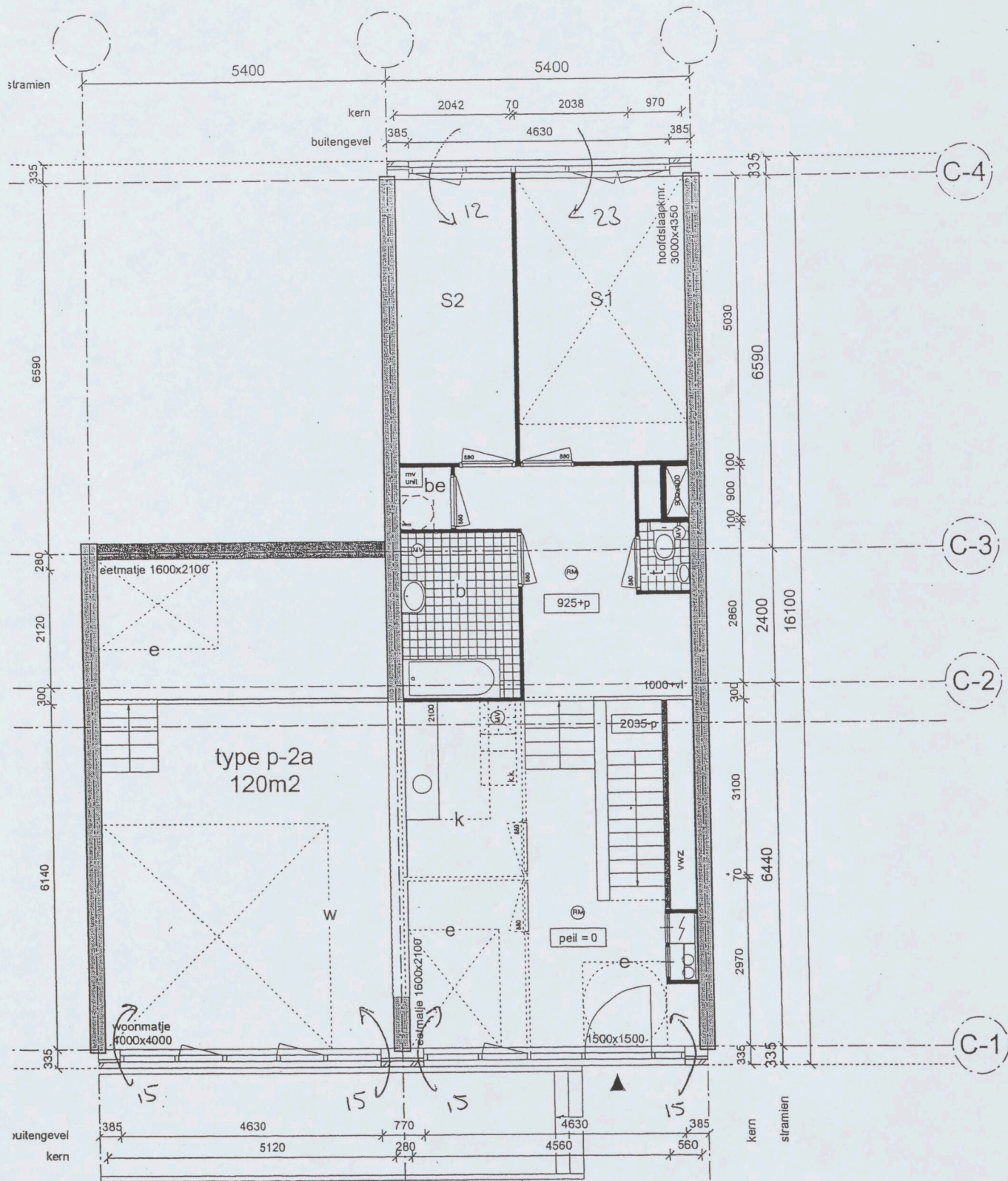
Type plintwoning 2a-nivo 0
