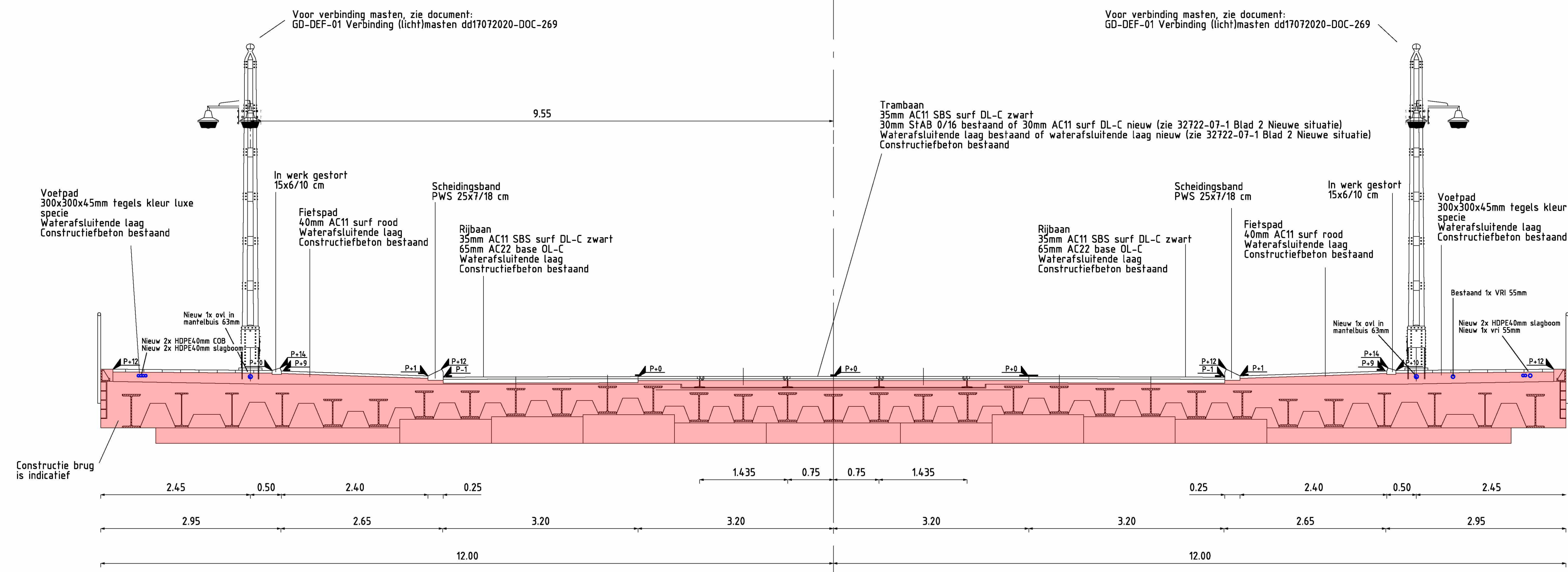
Dwarsprofiel E-E op aanbrug Nieuwe situatie schaal 1:50
