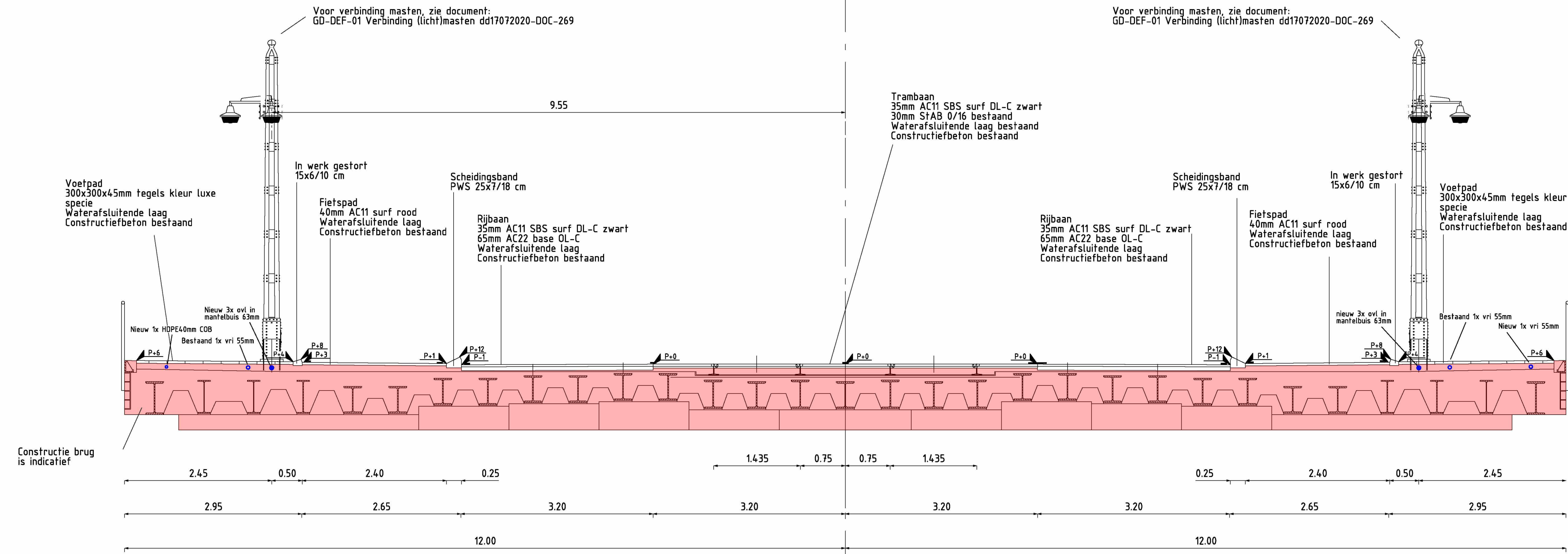
Dwarsprofiel G-G op aanbrug Nieuwe situatie schaal 1:50
