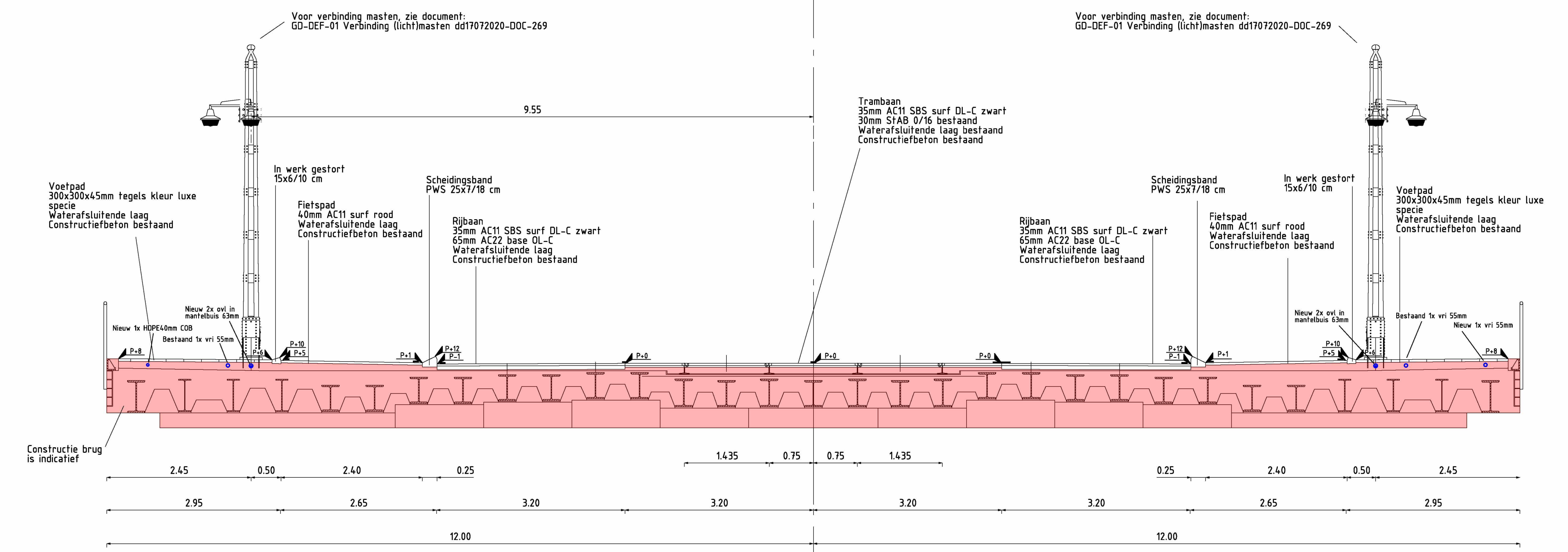
Dwarsprofiel F-F op aanbrug Nieuwe situatie schaal 1:50
