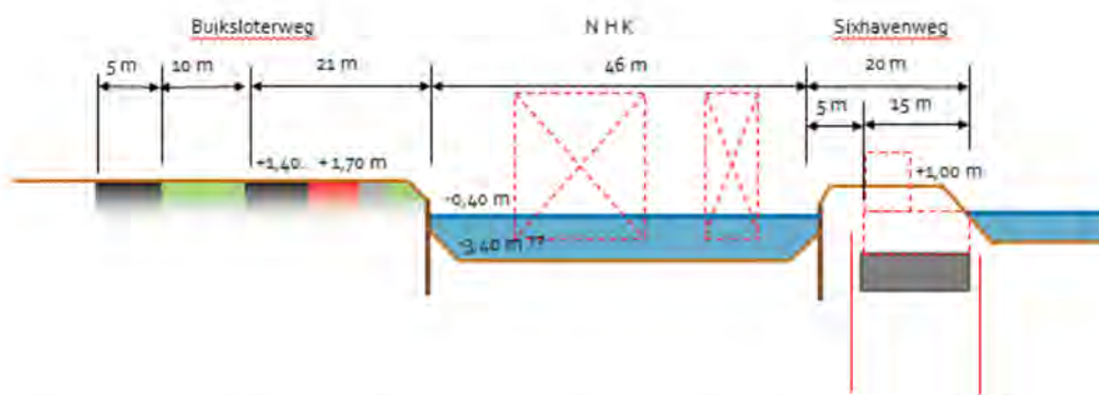
Doorsnede van Buiksloterweg-Noordhollandsch kanaal- Sixhavenweg
