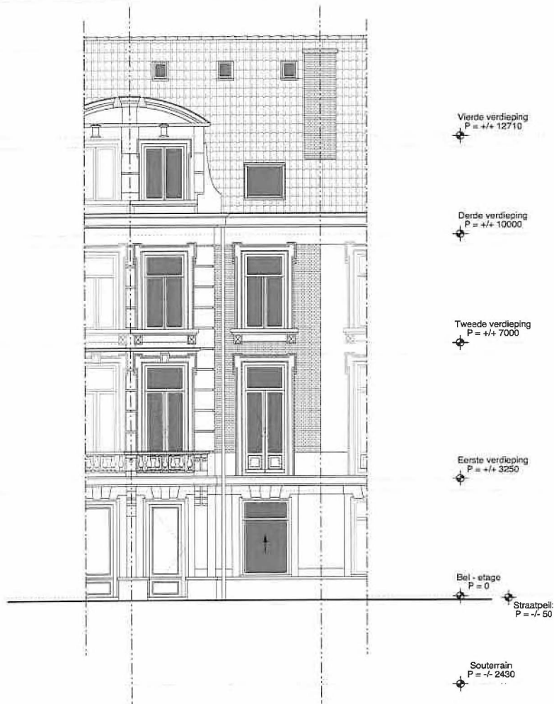
VOORGEVEL BESTAAND GEEN WIJZIGINGEN
