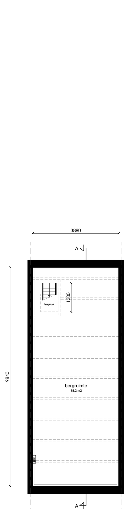
Kelder
