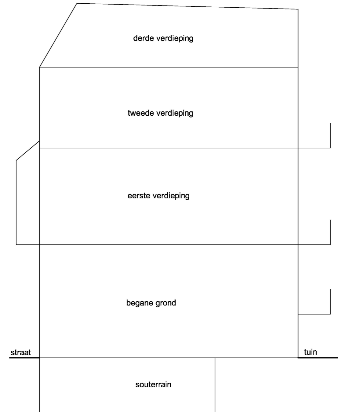
Doorsnede schaal 1:100
