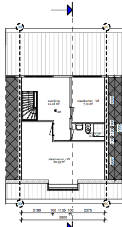
3e verdieping
