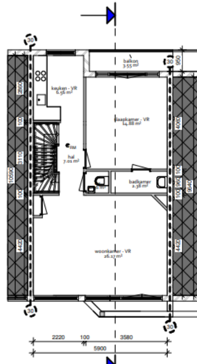
2e verdieping
