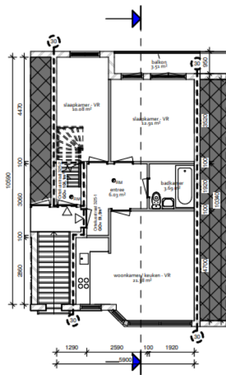
1e verdieping
