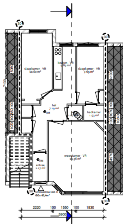
Begane grond
