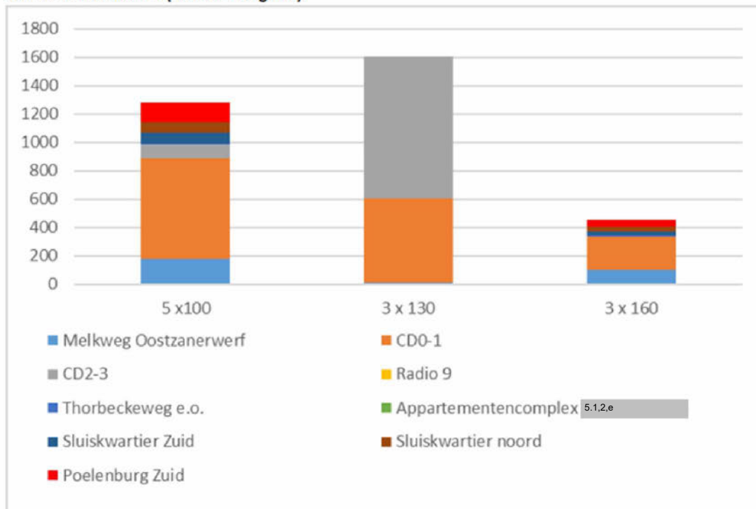
Figuur 5 Aantal ernstig gehinderden in gebieden met woningbouwplannen, als gevolg van geluidsproductie van de windturbines (zonder mitigatie).
