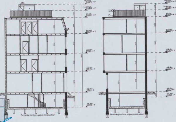
DOORSNEDE A-A Nieuwe situatie
