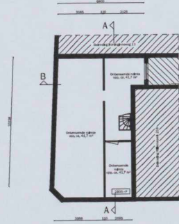
KELDER Willemsparking 2204a Bestaande situatie
