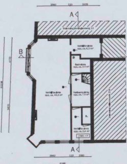
TWEDE VERDIEPING Willemsparking 2204 Bestaande situatie
