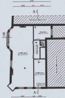
EERSTE VERDIEPING Willemsparking 2204 Nieuwe situatie
