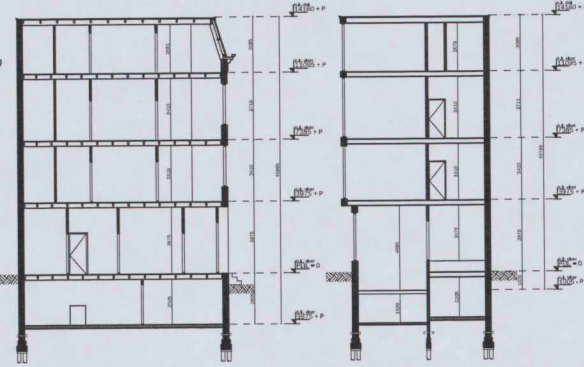
DOORSNEDE A-A Bestaande situatie
