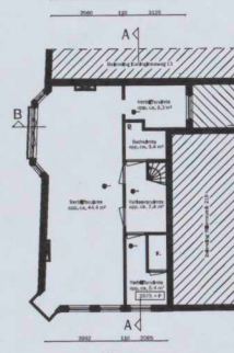
EERSTE VERDIEPING Willemsparking 2204 Bestaande situatie
