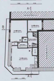
DERDE VERDIEPING Willemsparking 2204b Nieuwe situatie
