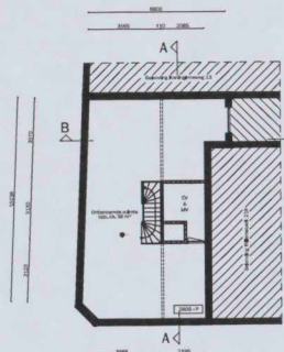
KELDER Willemsparking 2204a Nieuwe situatie
