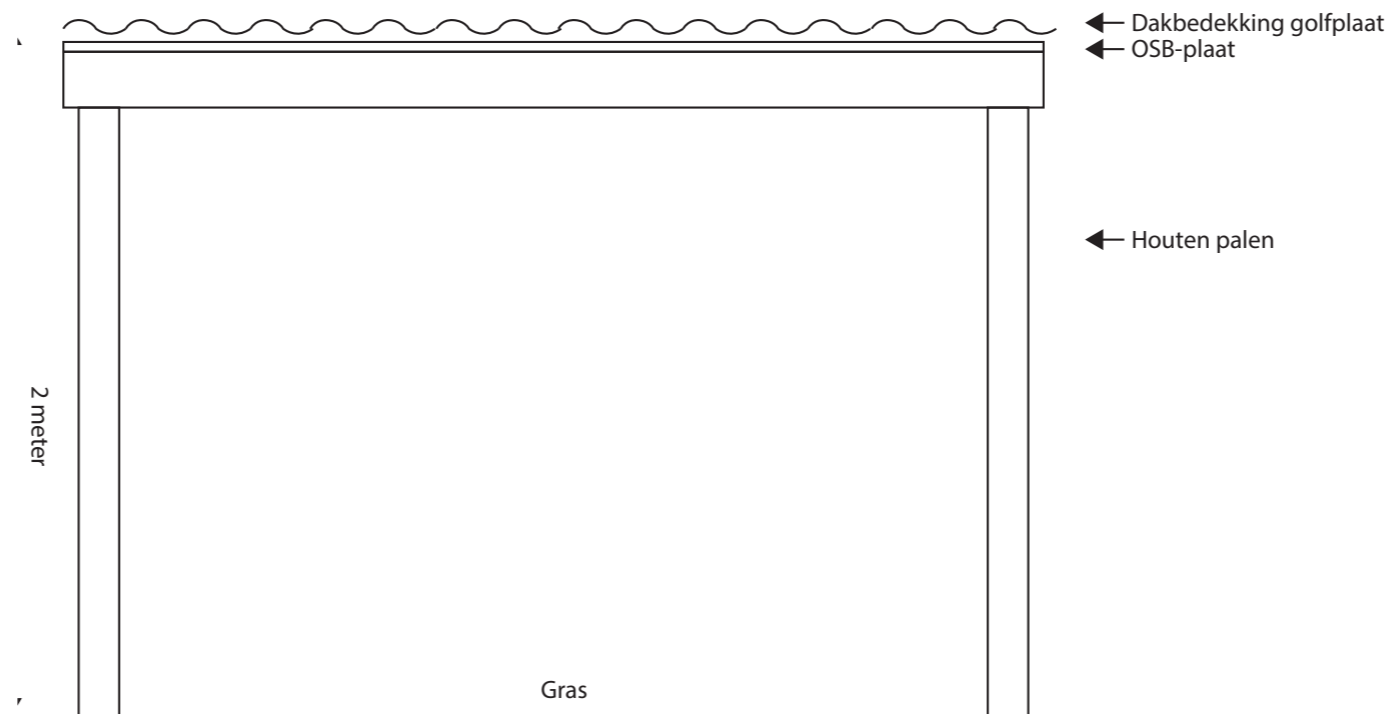
Voorraanzicht
