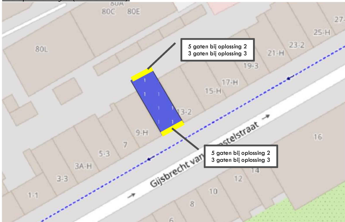
Figuur 12 – kelder is grondwaterneutraal bij toepassen maatregelen langs gevels welke geel zijn (voor alle oplosrichtingen).
