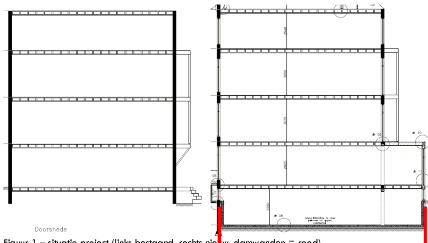
Figuur 1 – situatie project (links bestaand, rechts nieuw, damwanden = rood)
