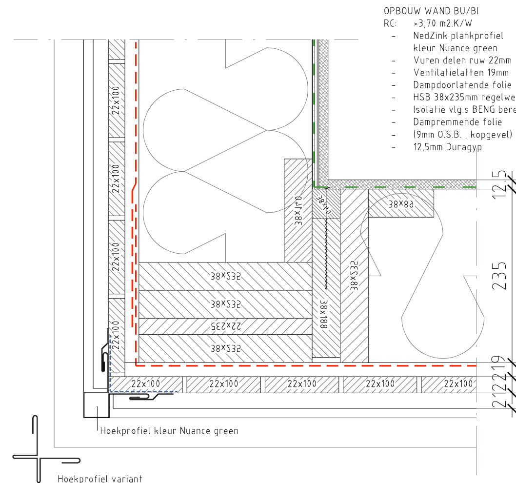
Hoekprofiel variant
