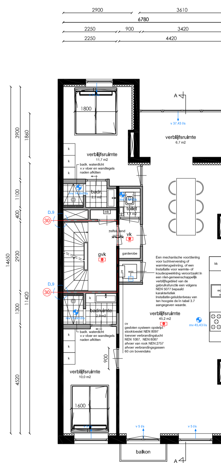
Tweede verdieping
