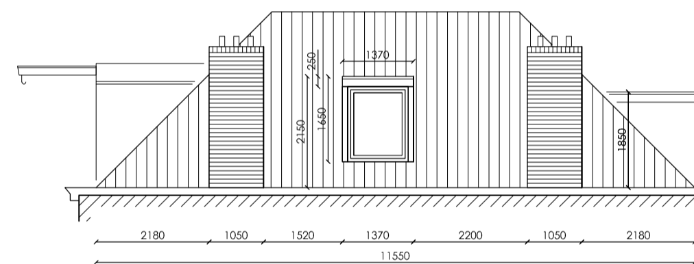
Rechter zijgevel
