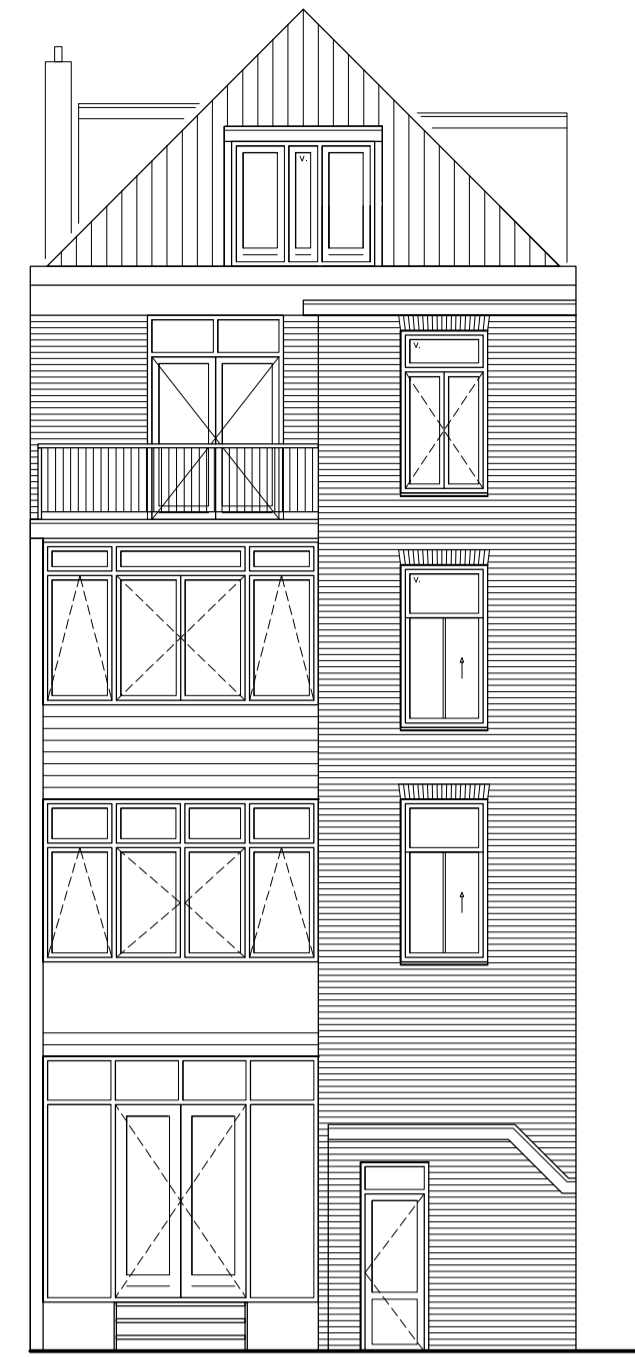
Achtergevel
