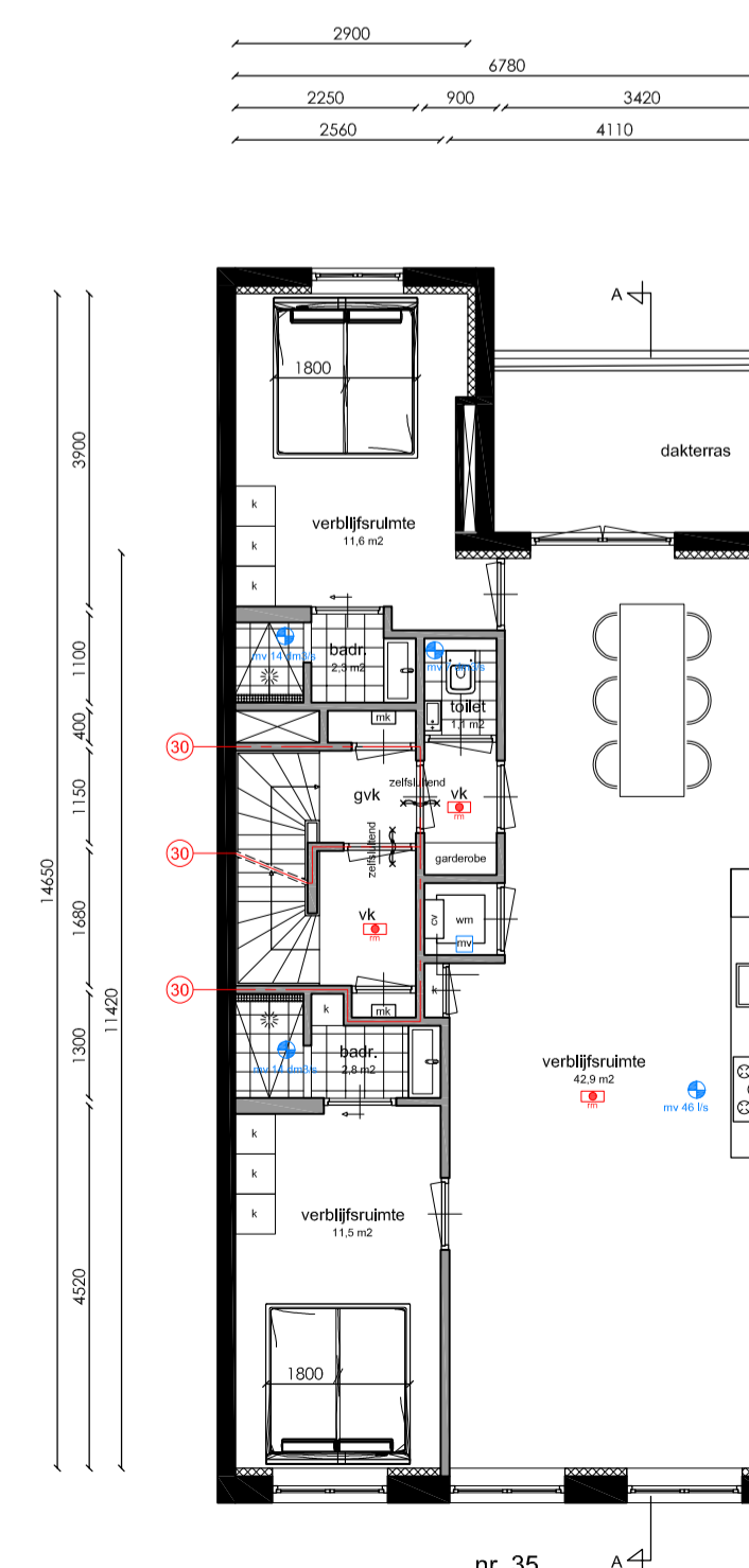
Derde verdieping
