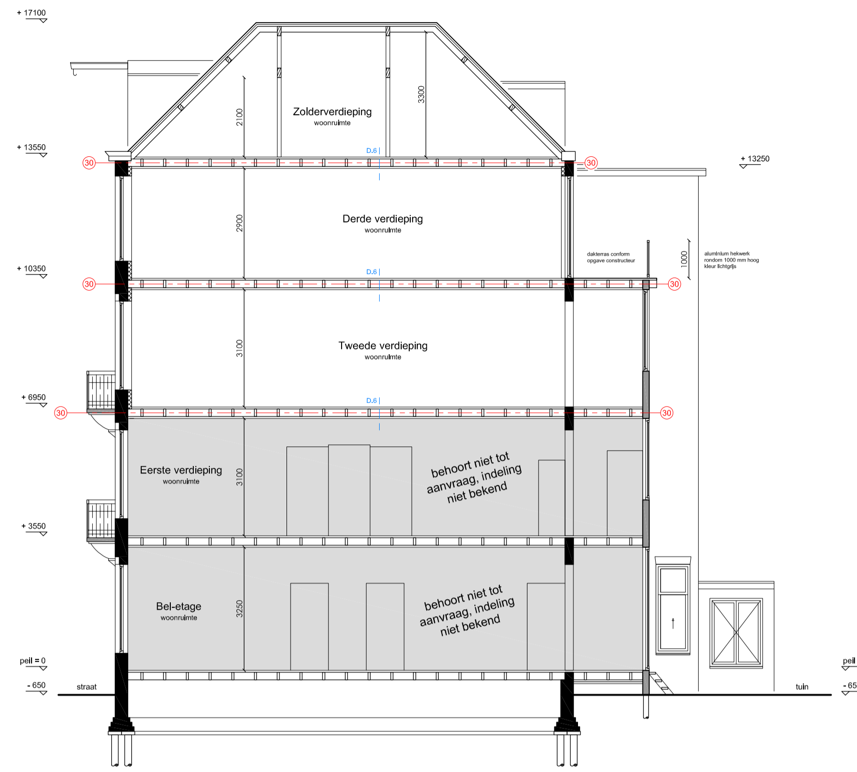
Doorsnede A-A
