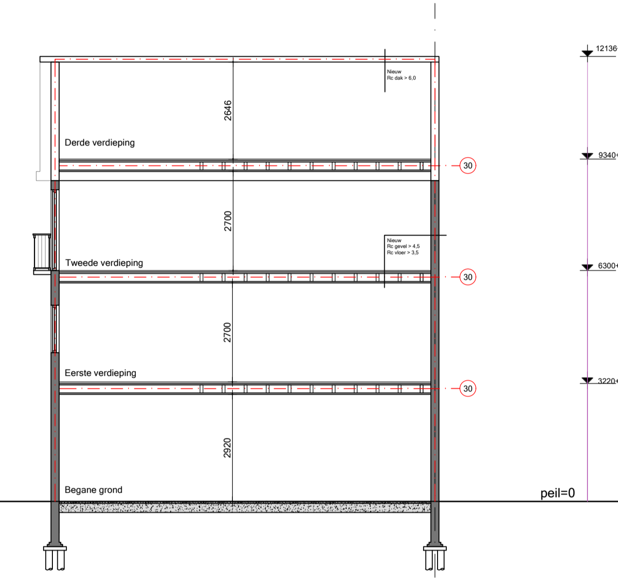
Doorsnede A-A
