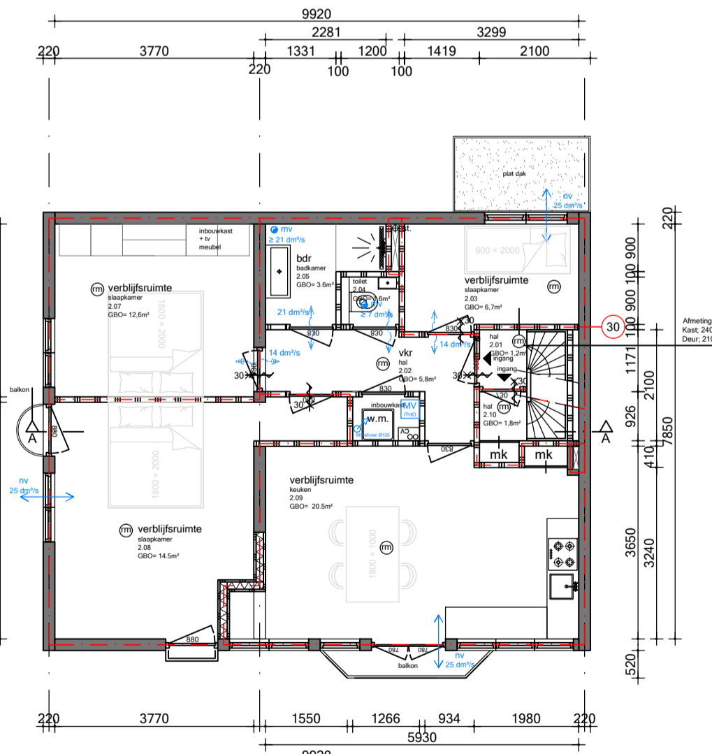
Tweede verdieping
