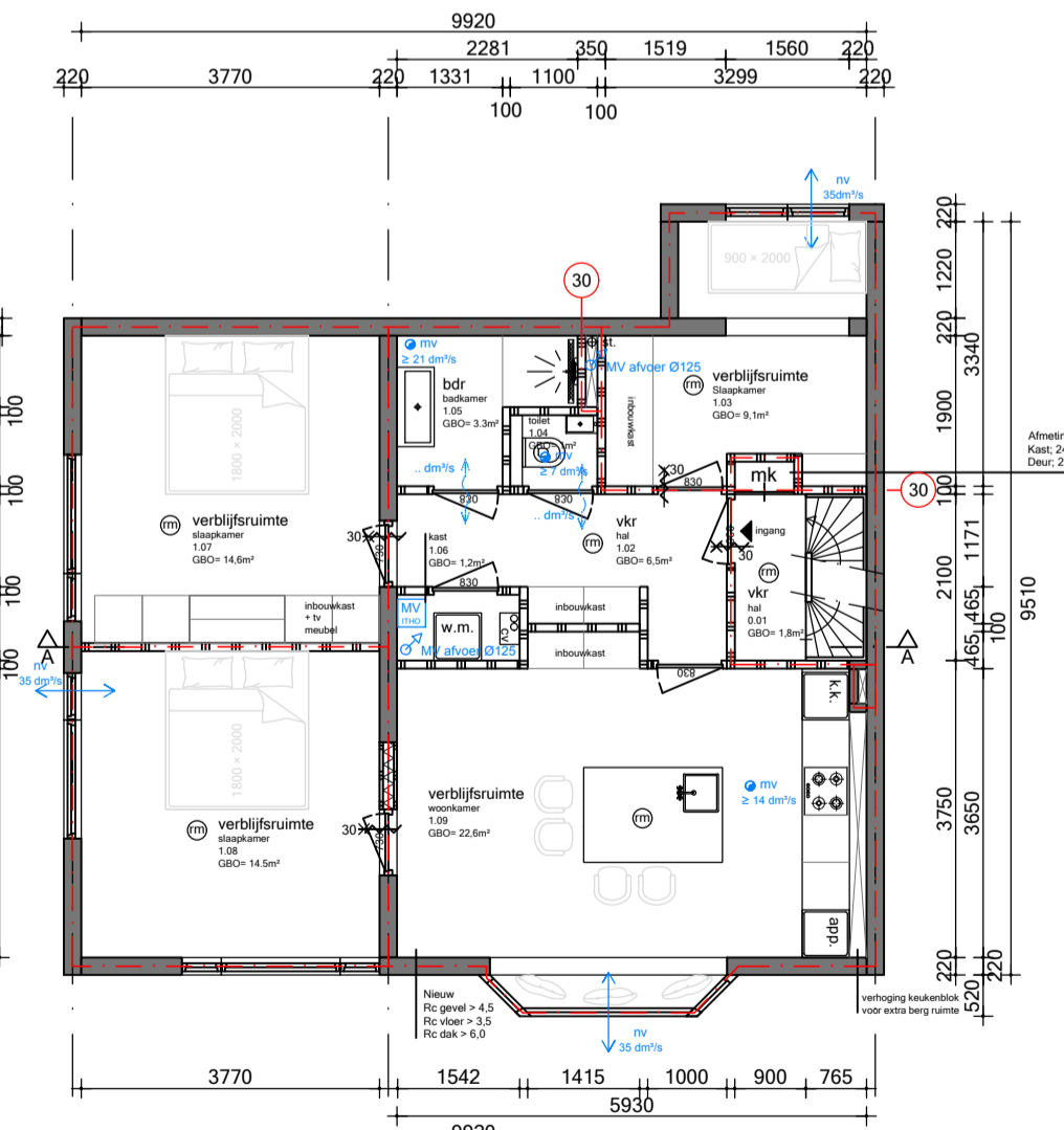
Eerste verdieping
