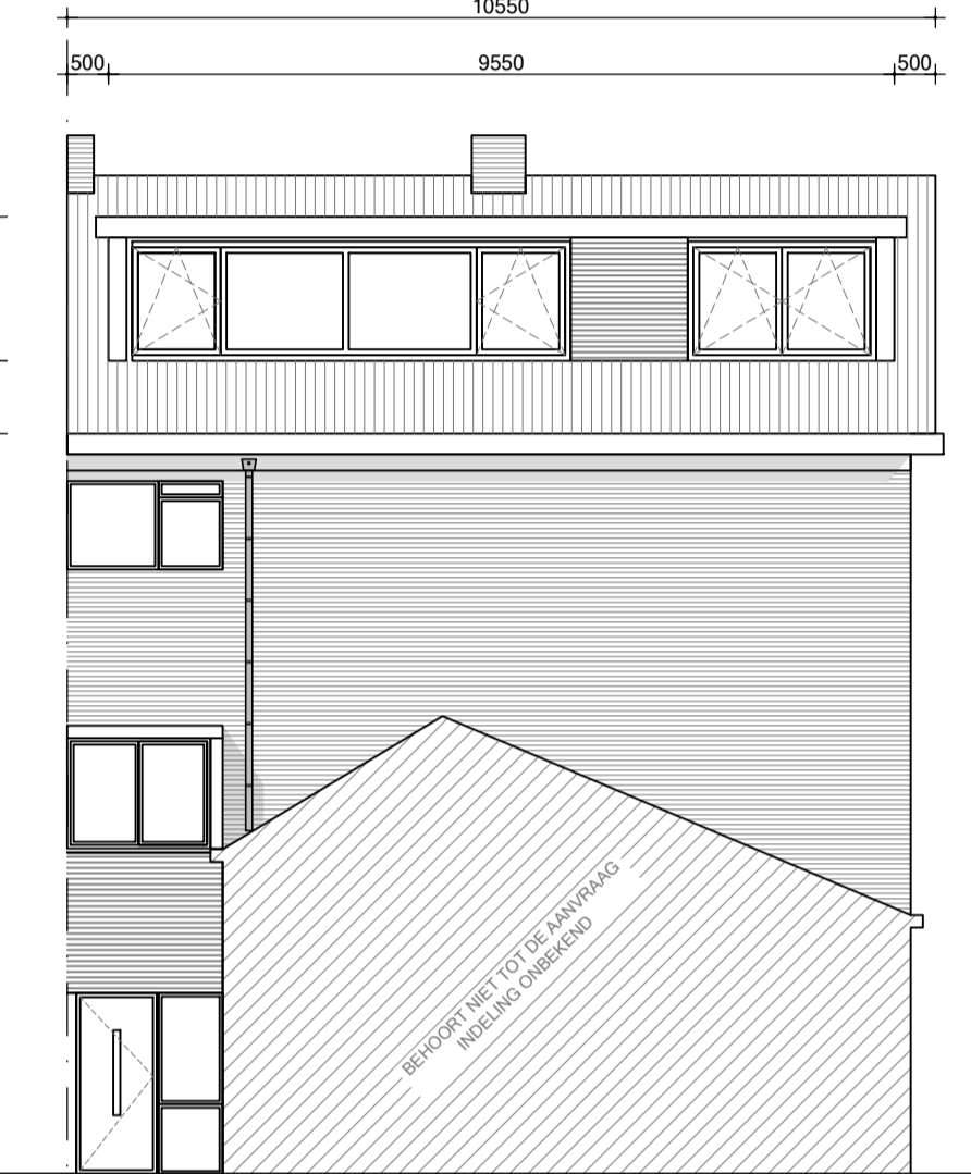
Achter aanzicht
