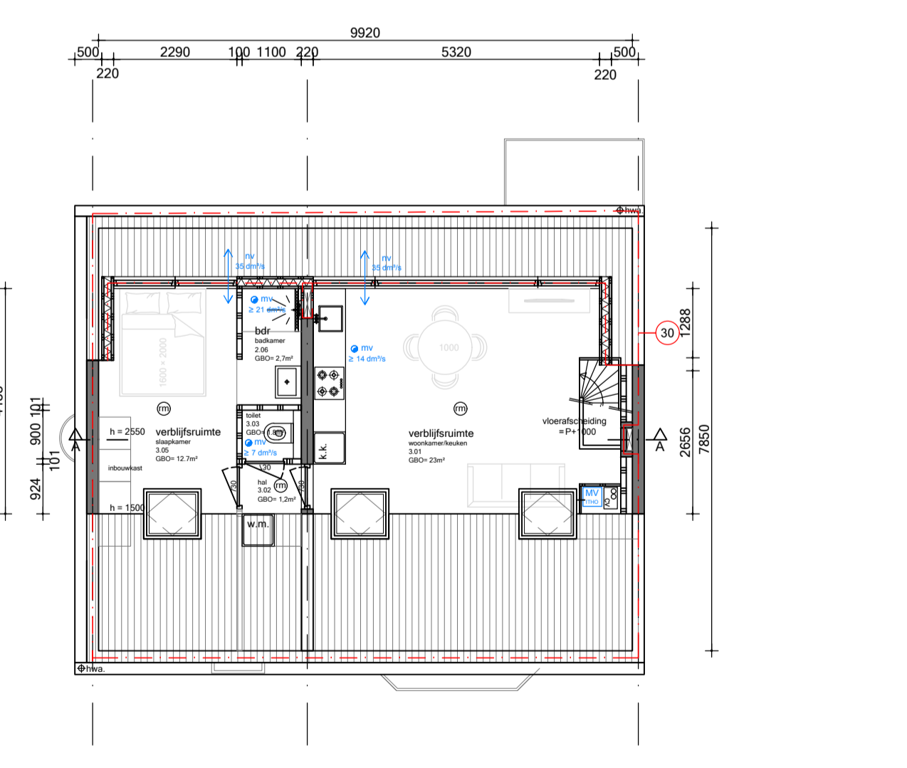
Derde verdieping
