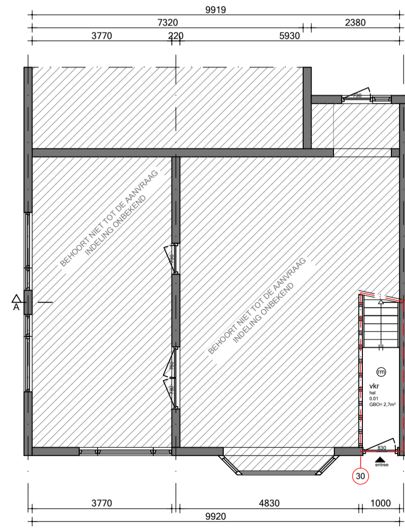
Begane grond
