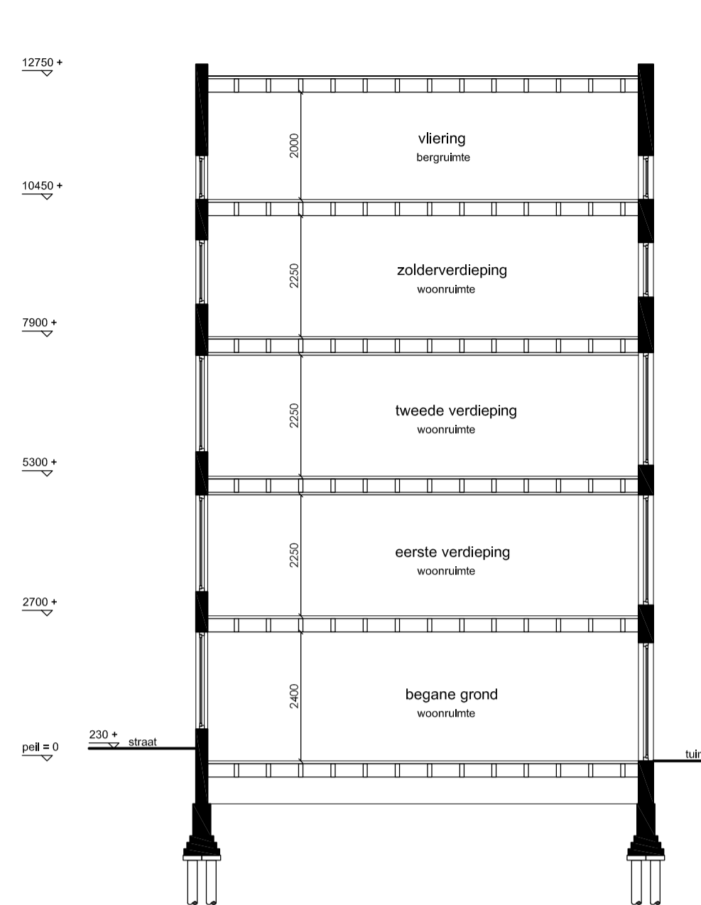
Doorsnede A-A
