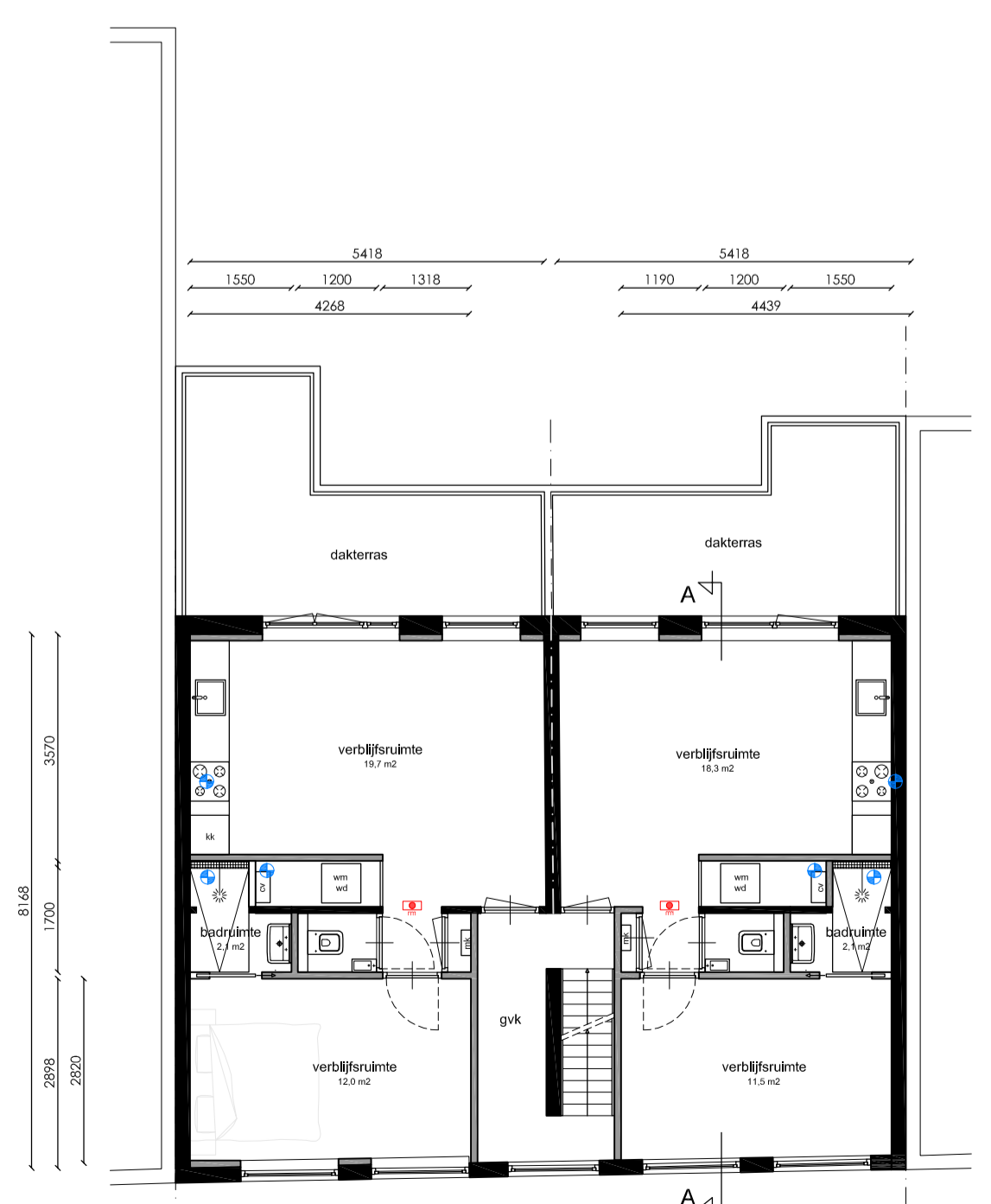
Eerste verdieping
