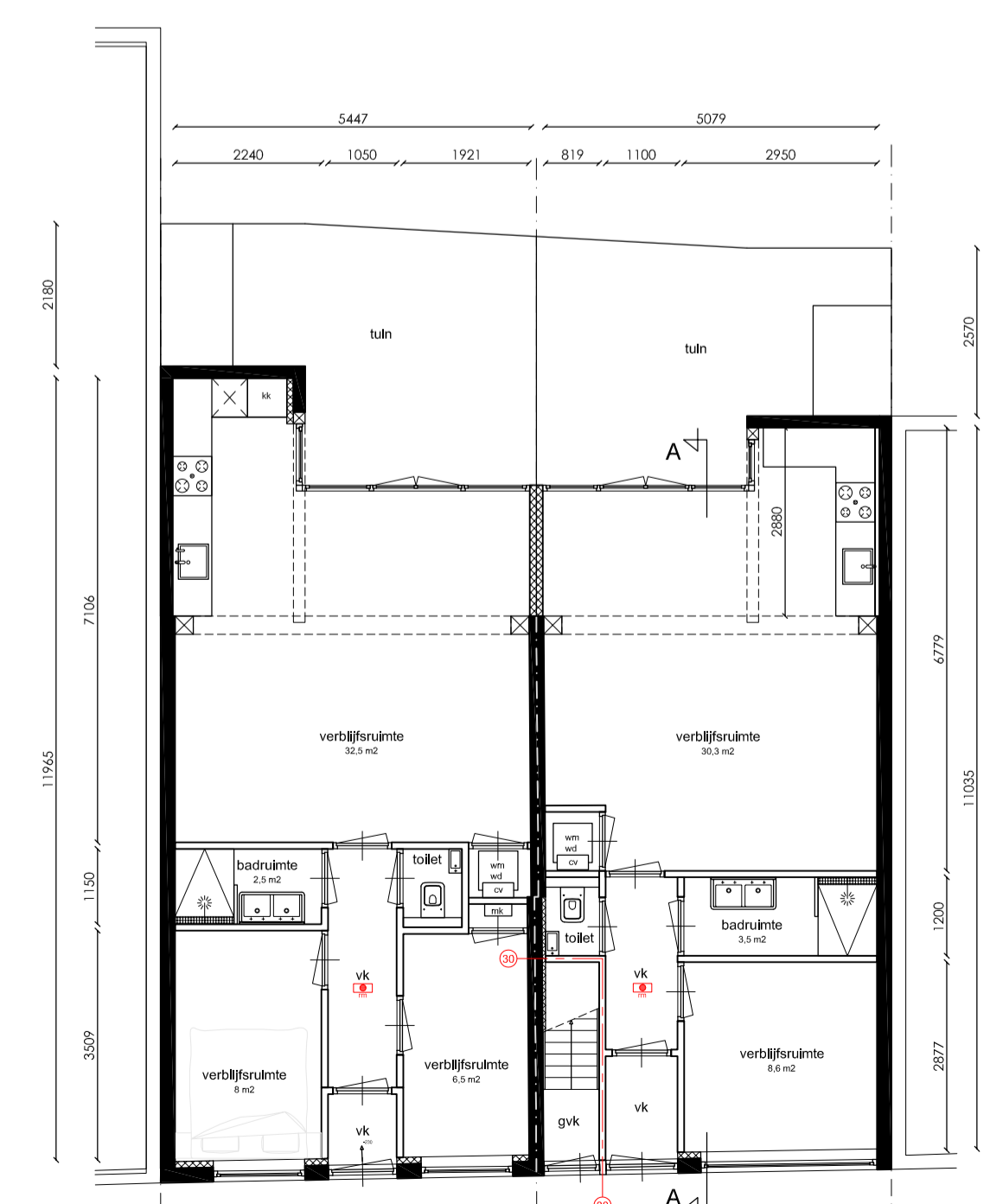
Begane grond
