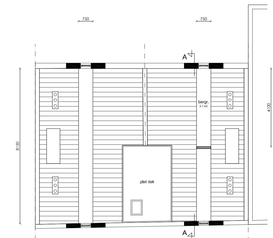
Vliering
