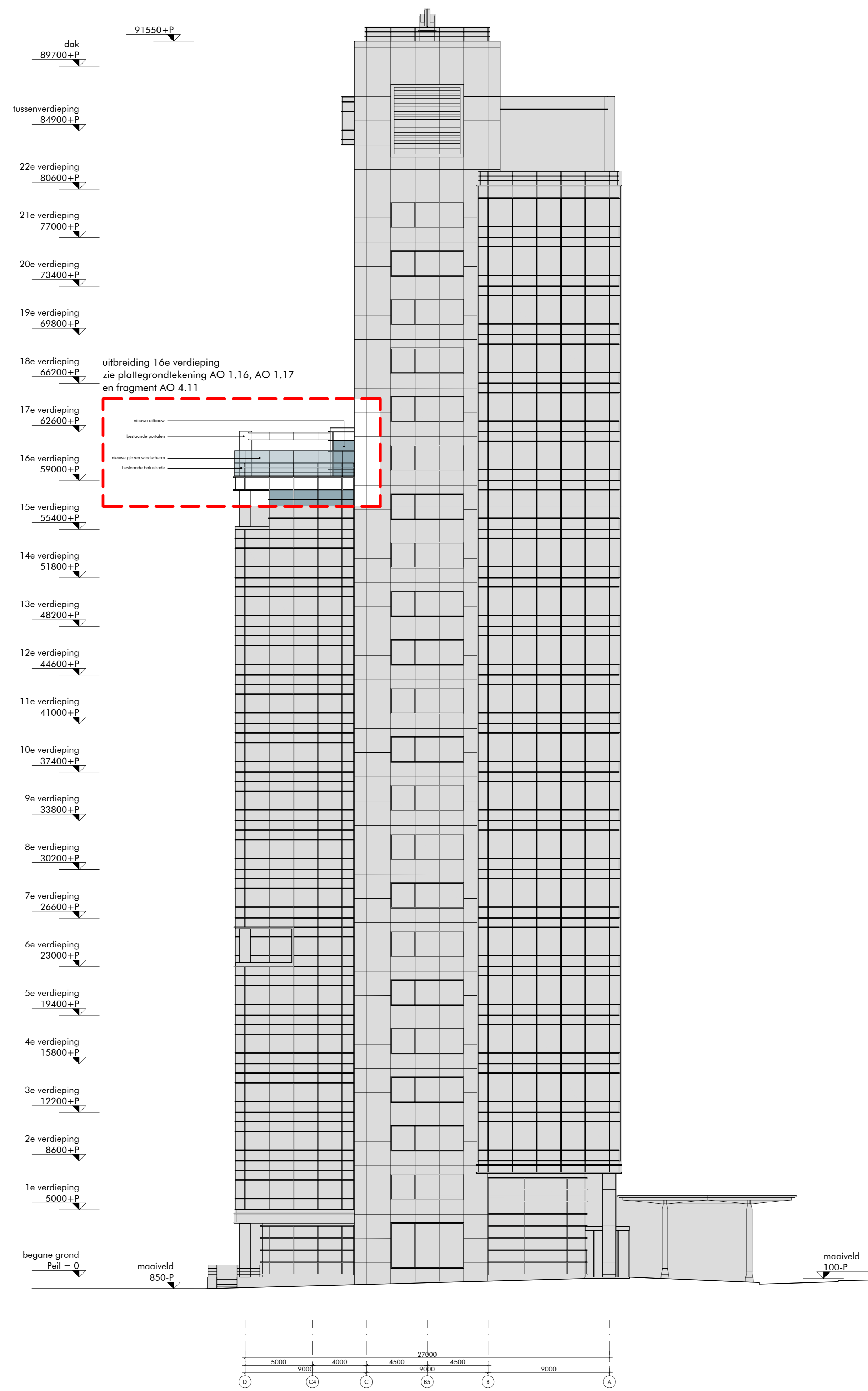
zuidgevel
