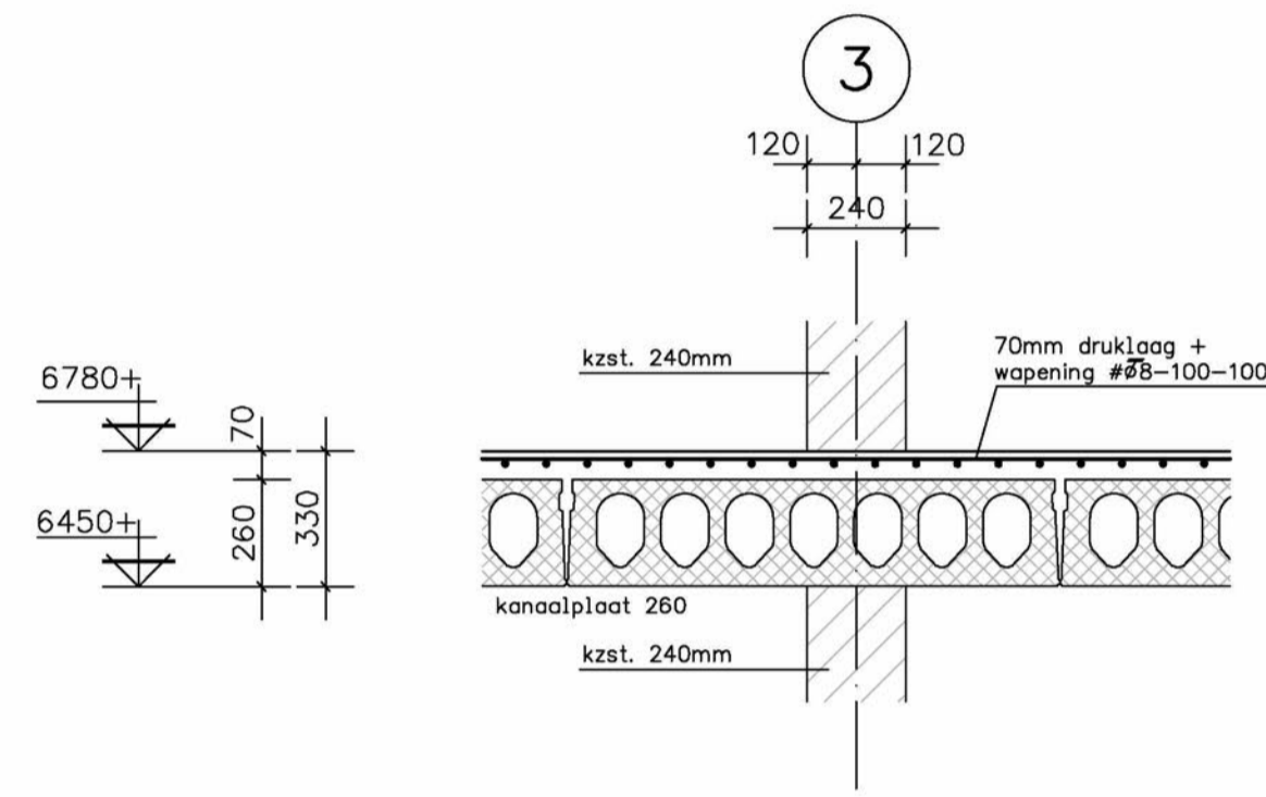
DOORSNEDE G-G.
