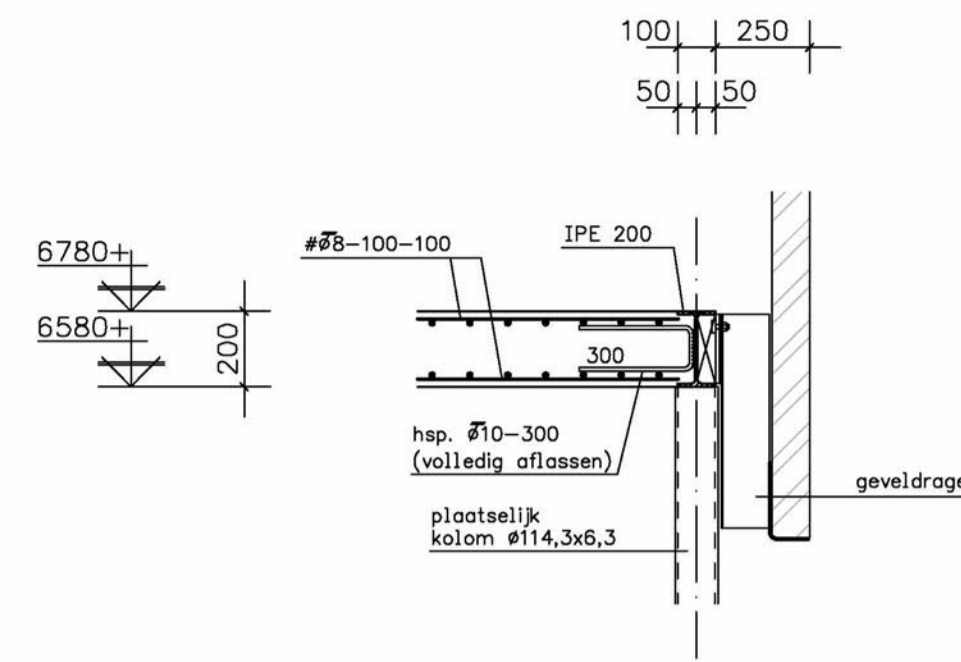
DOORSNEDE C-C.
