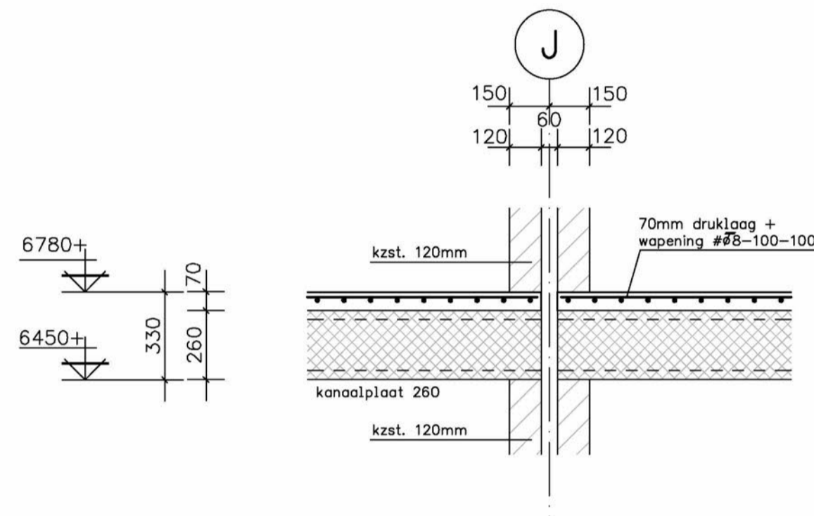
DOORSNEDE F1-F1.
