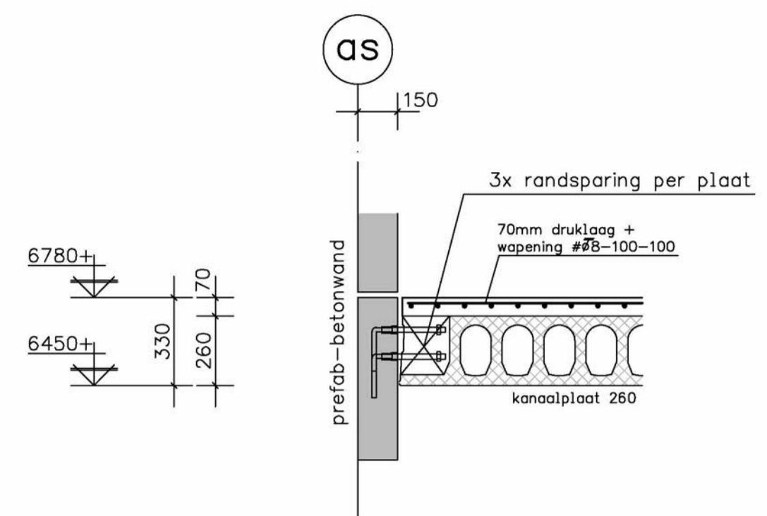
DOORSNEDE E-E.
