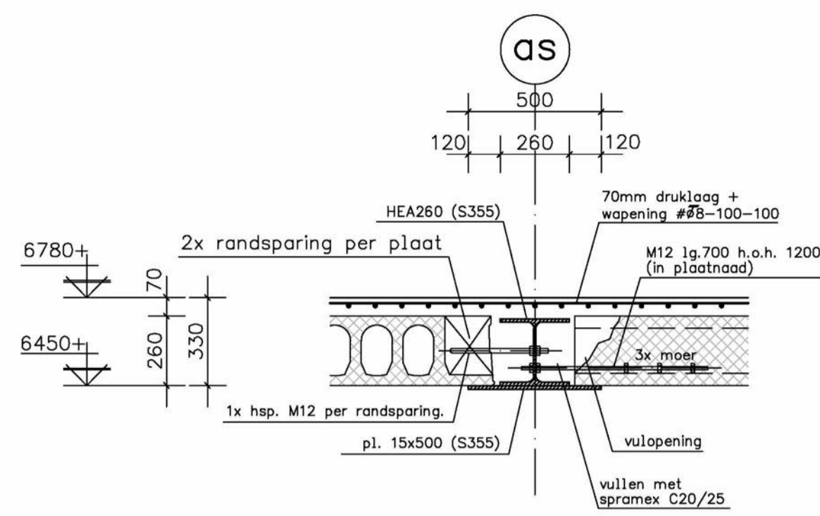
DOORSNEDE A-A.
