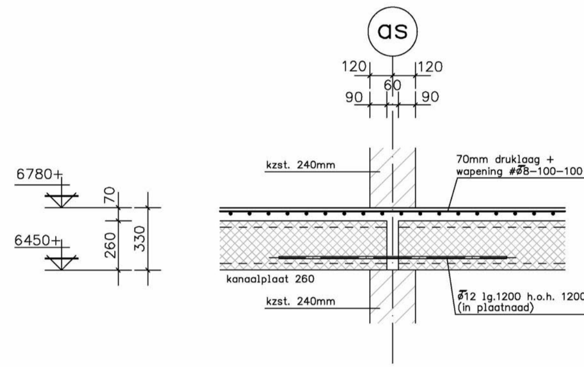
DOORSNEDE F-F.
