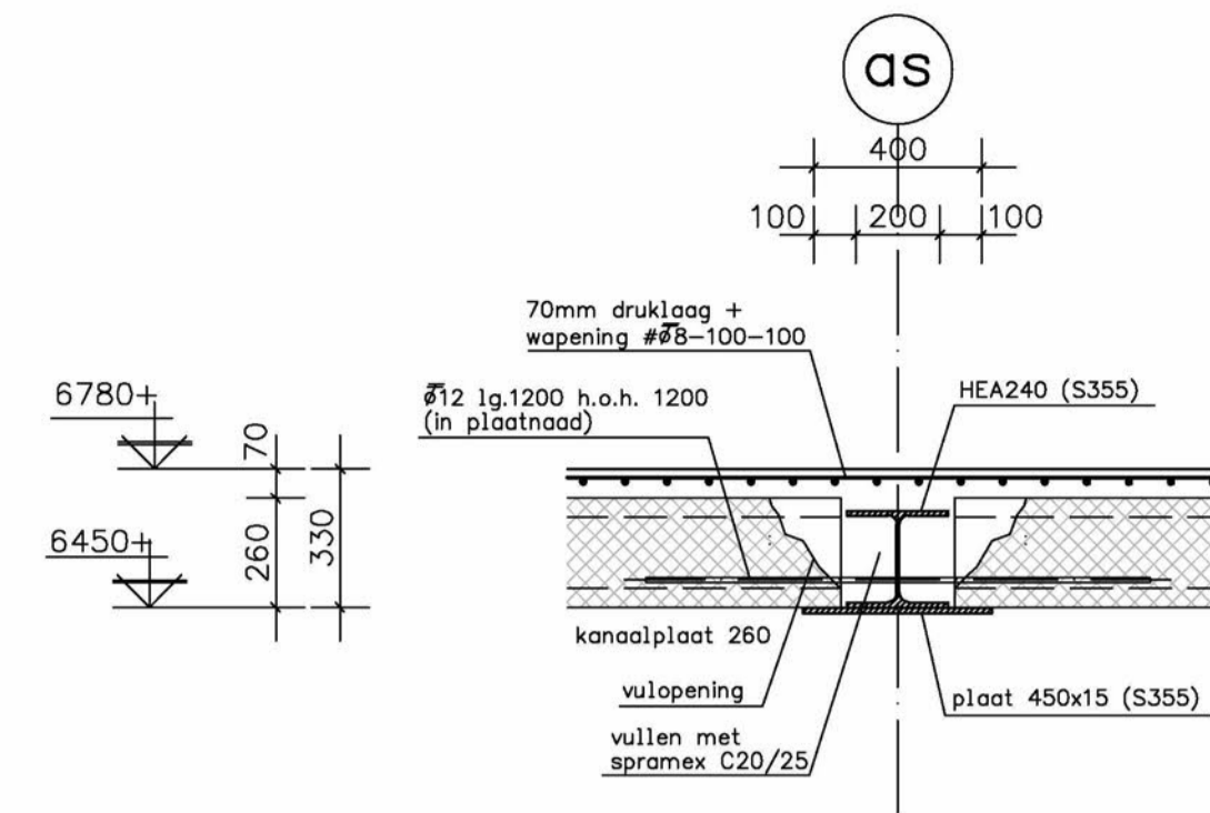
DOORSNEDE D-D.
