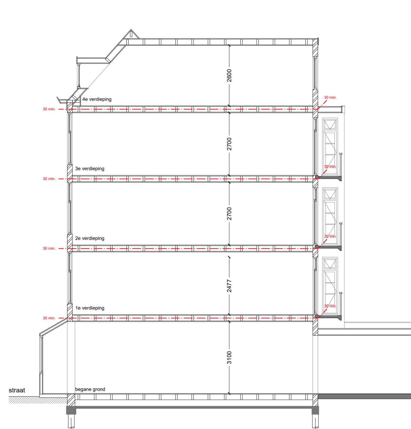
DOORSNEDE a-a
