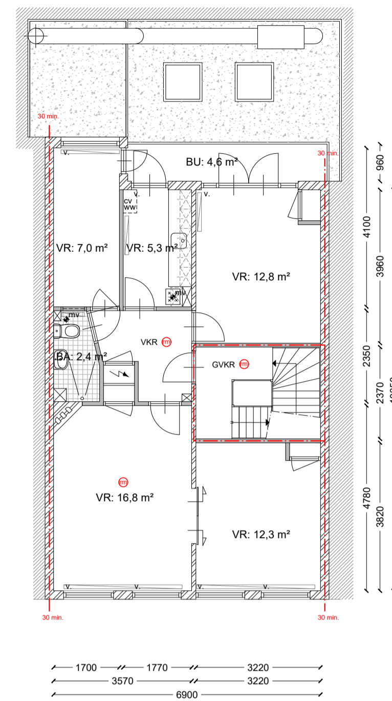
1e VERDIEPING
