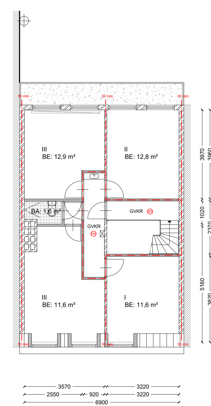
4e VERDIEPING
