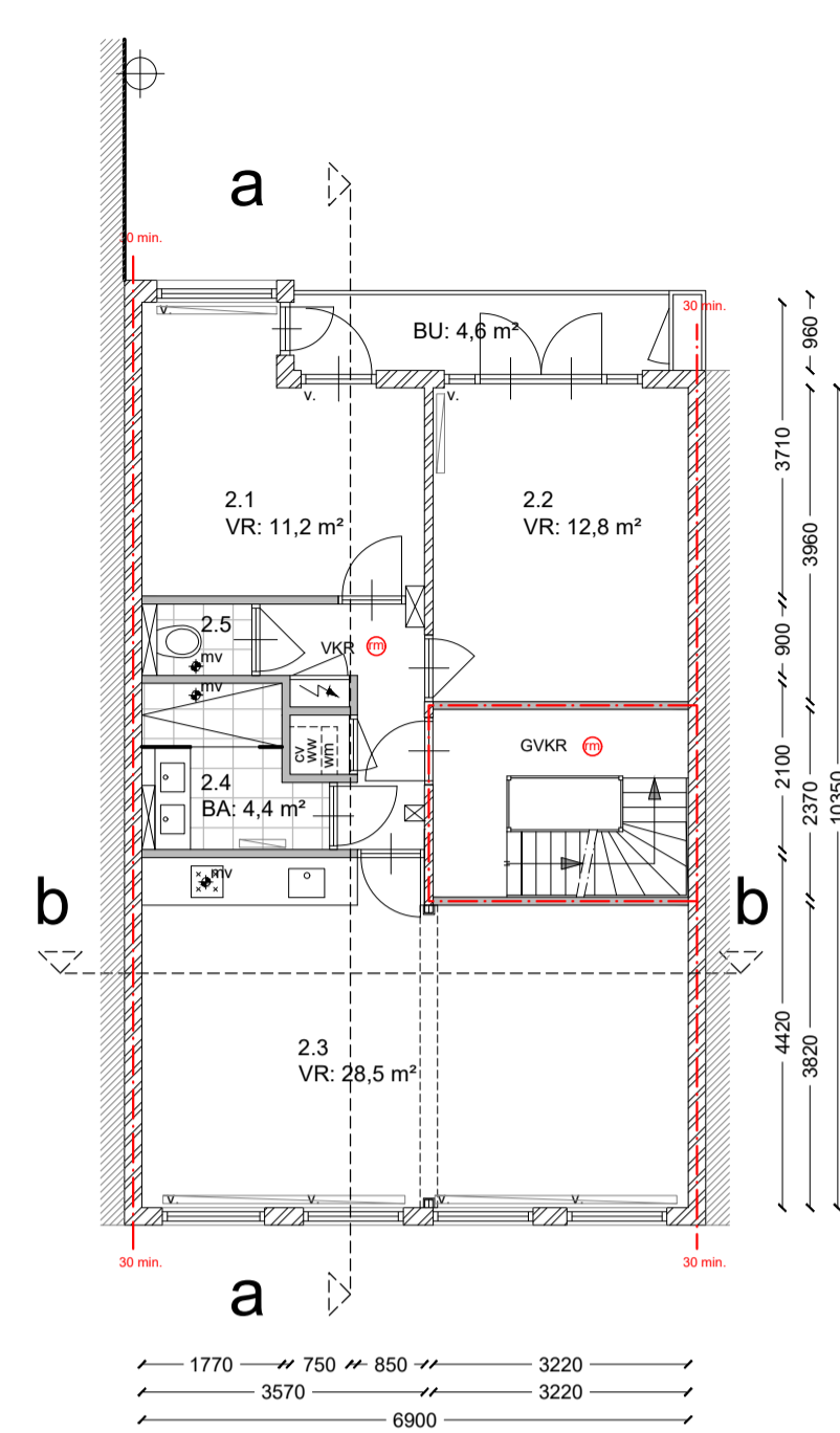
2e VERDIEPING
