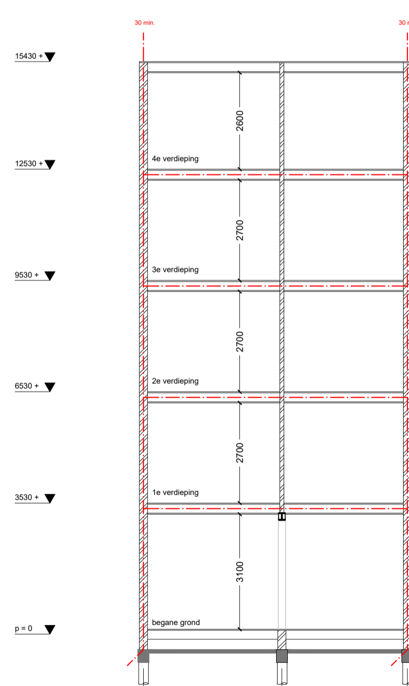
DOORSNEDE b-b
