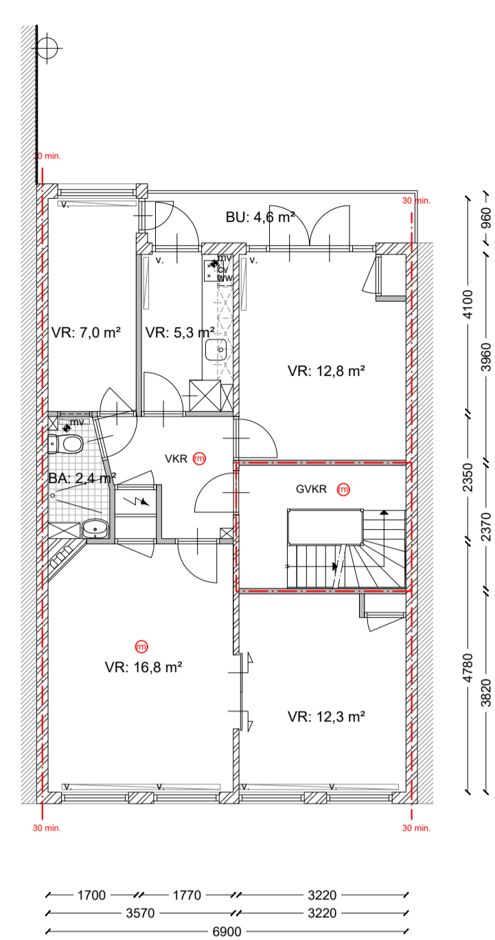
3e VERDIEPING
