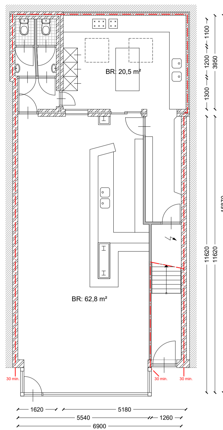
BEGANE GROND
