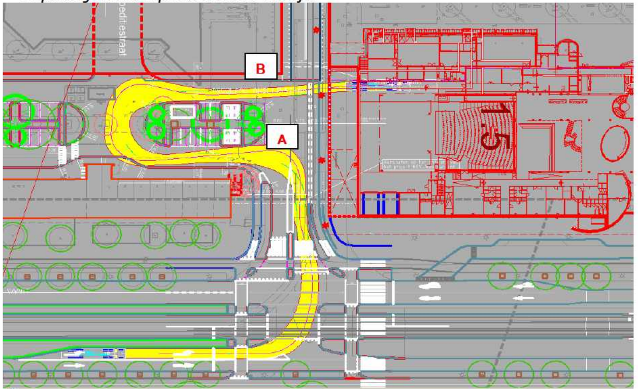
Afbeelding situatie 2a, laad en losdok aan de zijde van N. Anslinstraat (vooruitrijden in de dok)
