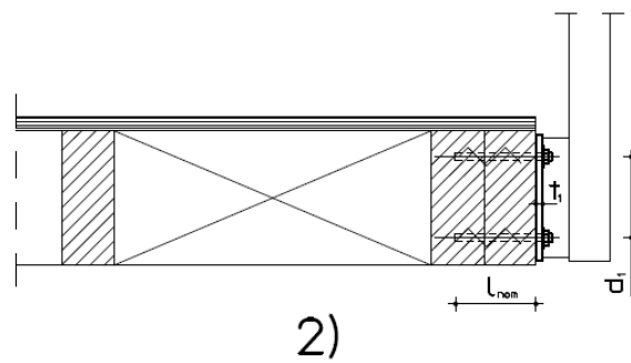
Twee varianten voor verankering van het hekwerk.
