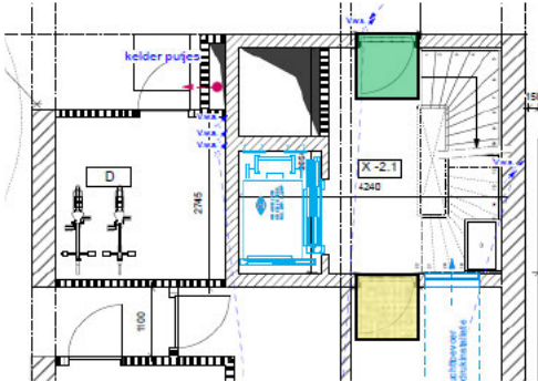
Kelder
