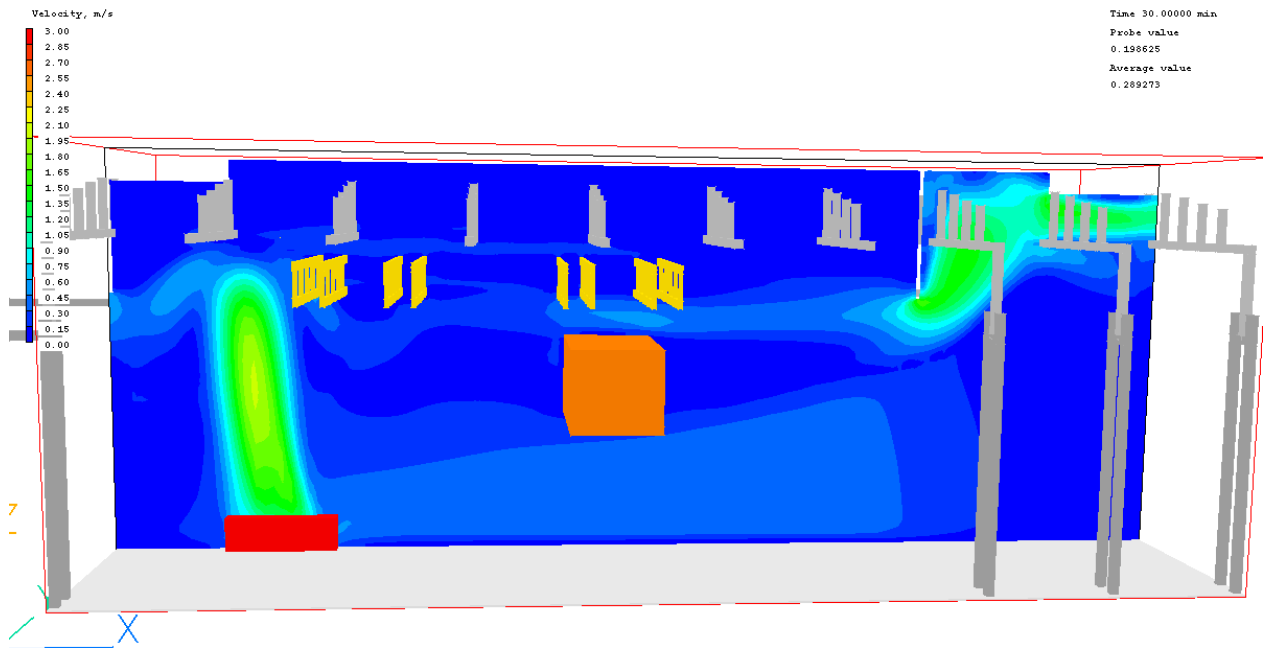
Figuur 121: Luchtsnelheden 30 minuten na aanvang brand, langsdoorsnede
