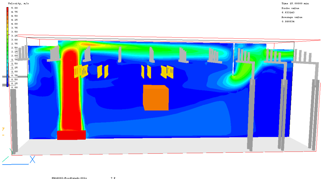
Figuur 109: Luchtsnelheden 15 minuten na aanvang brand, langdoorsnede
