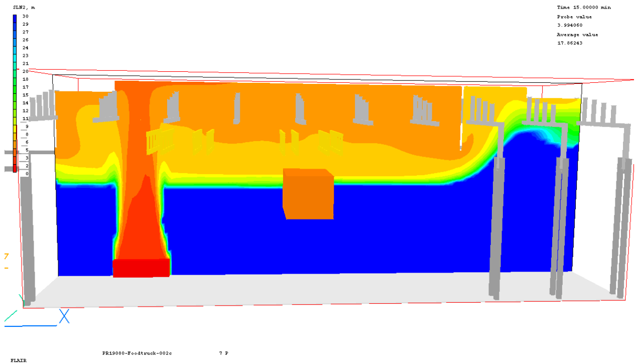
Figuur 110: Zichtlengte 15 minuten na aanvang brand, langdoorsnede
