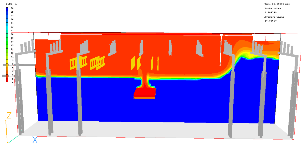
Figuur 214: Zichtlengte 20 minuten na aanvang brand, langdoorsnede
