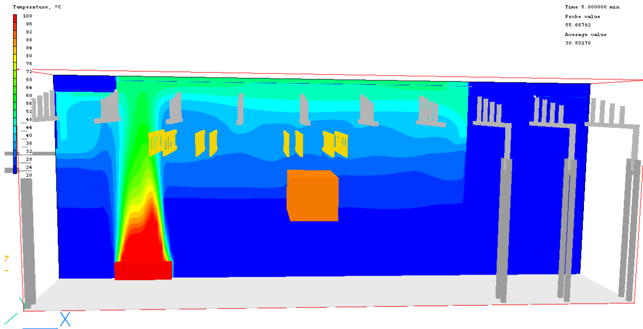
Figuur 103: Temperatuur 5 minuten na aanvang brand, langsdoorsnede
