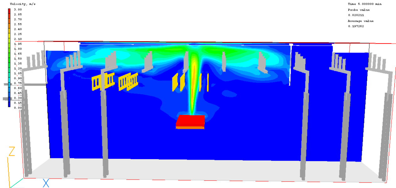
Figuur 201: Luchtsnelheden 5 minuten na aanvang brand, langsdoorsnede
