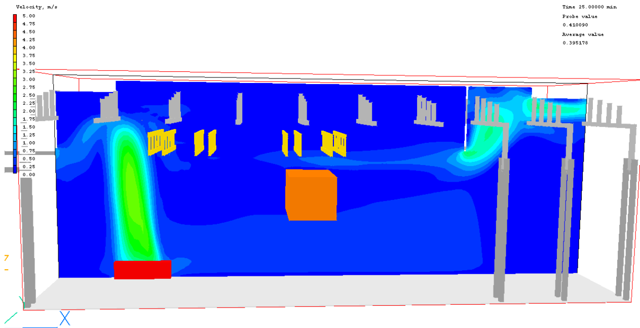
Figuur 117: Luchtsnelheden 25 minuten na aanvang brand, langdoorsnede
