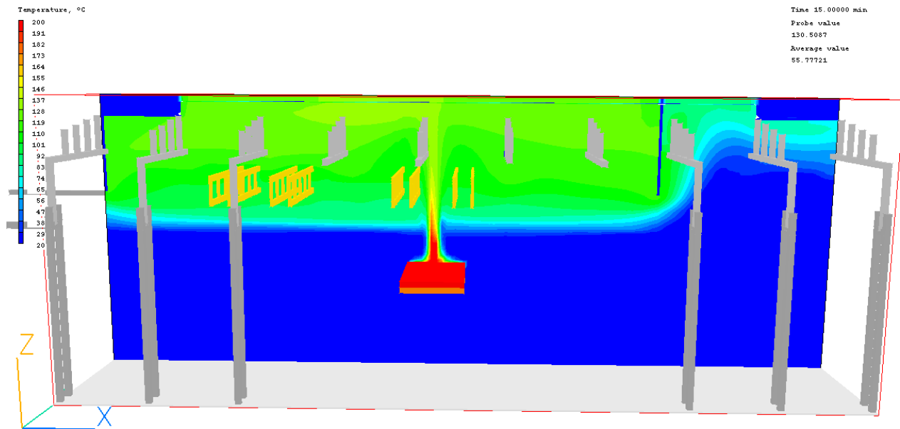
Figuur 211: Temperatuur 15 minuten na aanvang brand, langdoorsnede
