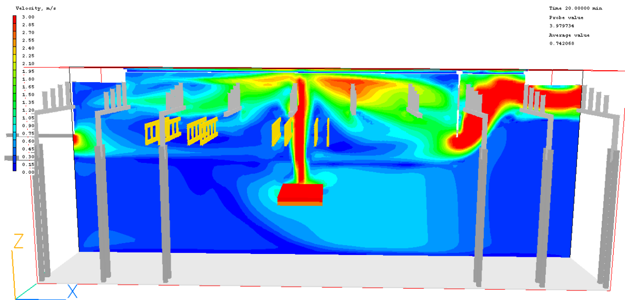
Figuur 213: Luchtsnelheden 20 minuten na aanvang brand, langdoorsnede
