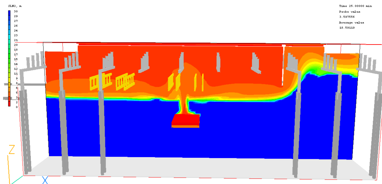
Figuur 218: Zichtlengte 25 minuten na aanvang brand, langdoorsnede
