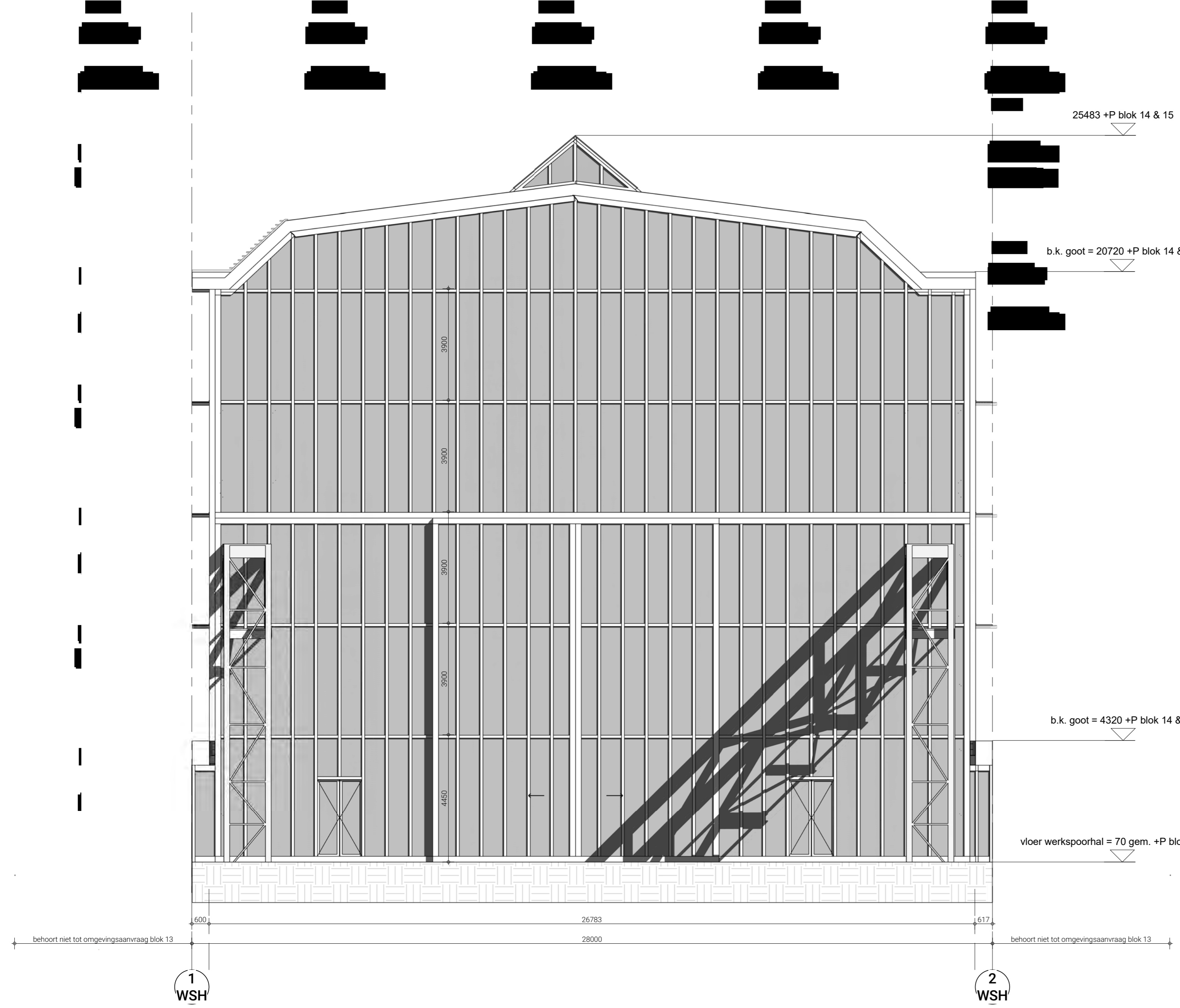
Zuidoostgevel 1:100
