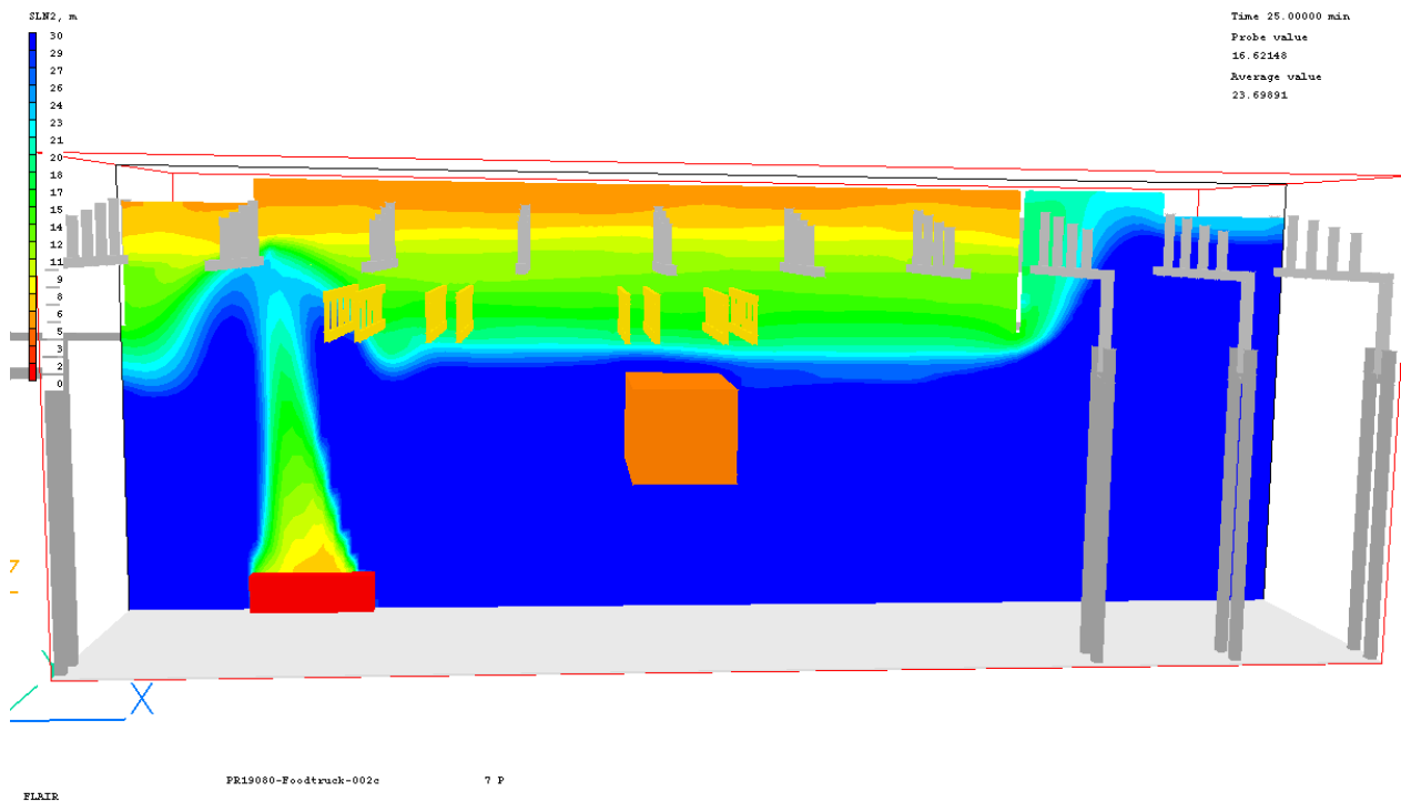
Figuur 118: Zichtlengte 25 minuten na aanvang brand, langdoorsnede
