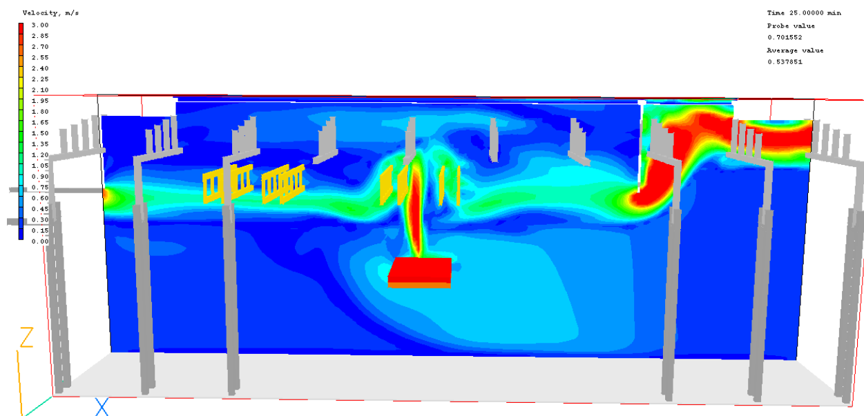
Figuur 217: Luchtsnelheden 25 minuten na aanvang brand, langdoorsnede
