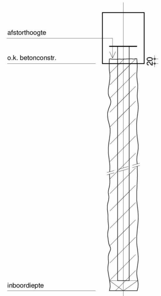
Algemeen detail paal In de grond gemaakte palen (Schroef injectiepalen)
