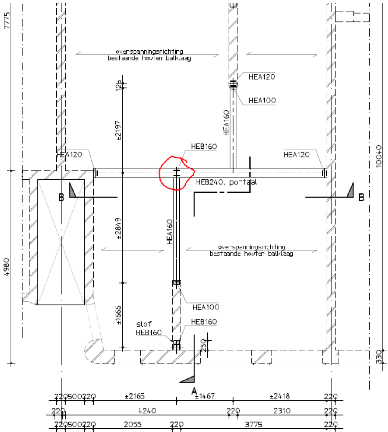
1e verdieping
