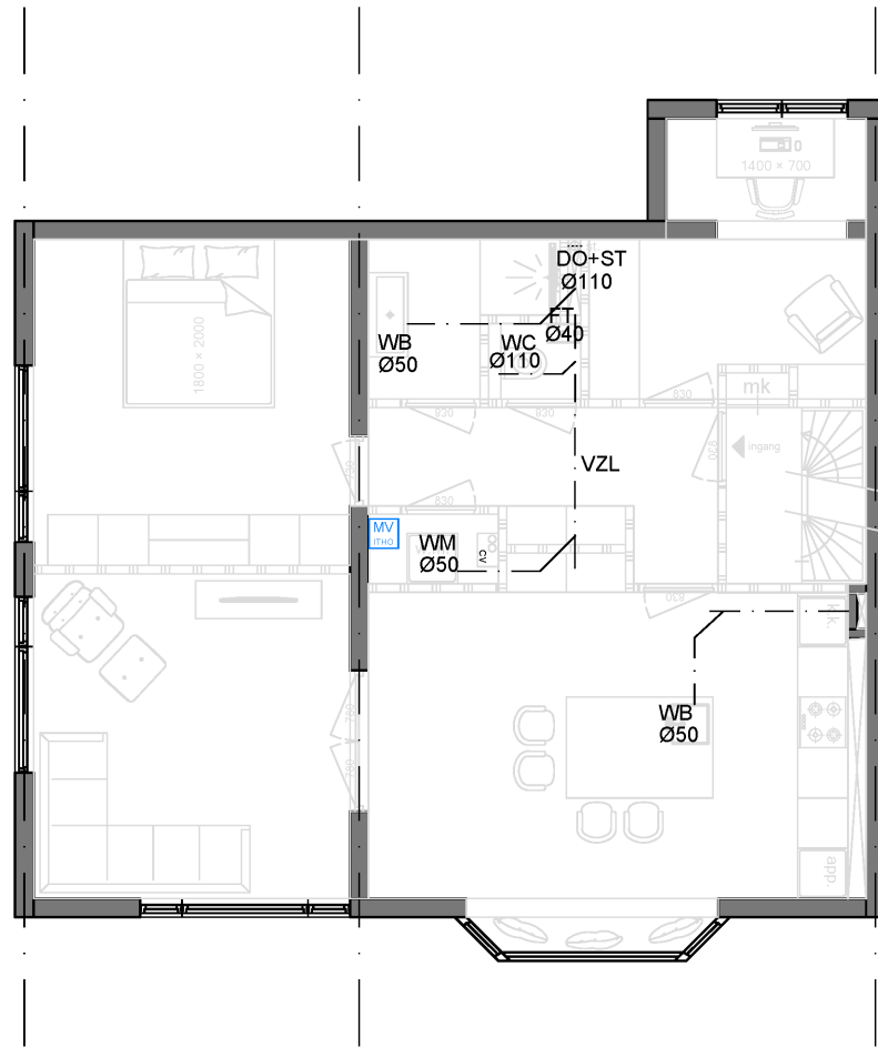
Eerste verdieping
