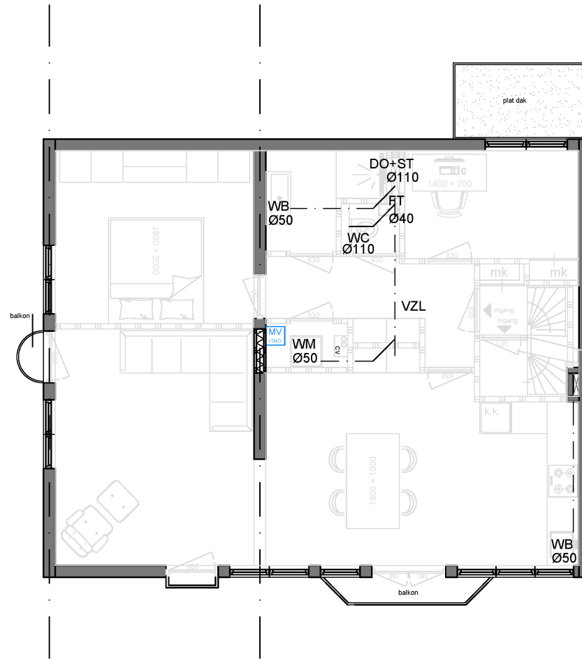
Tweede verdieping
