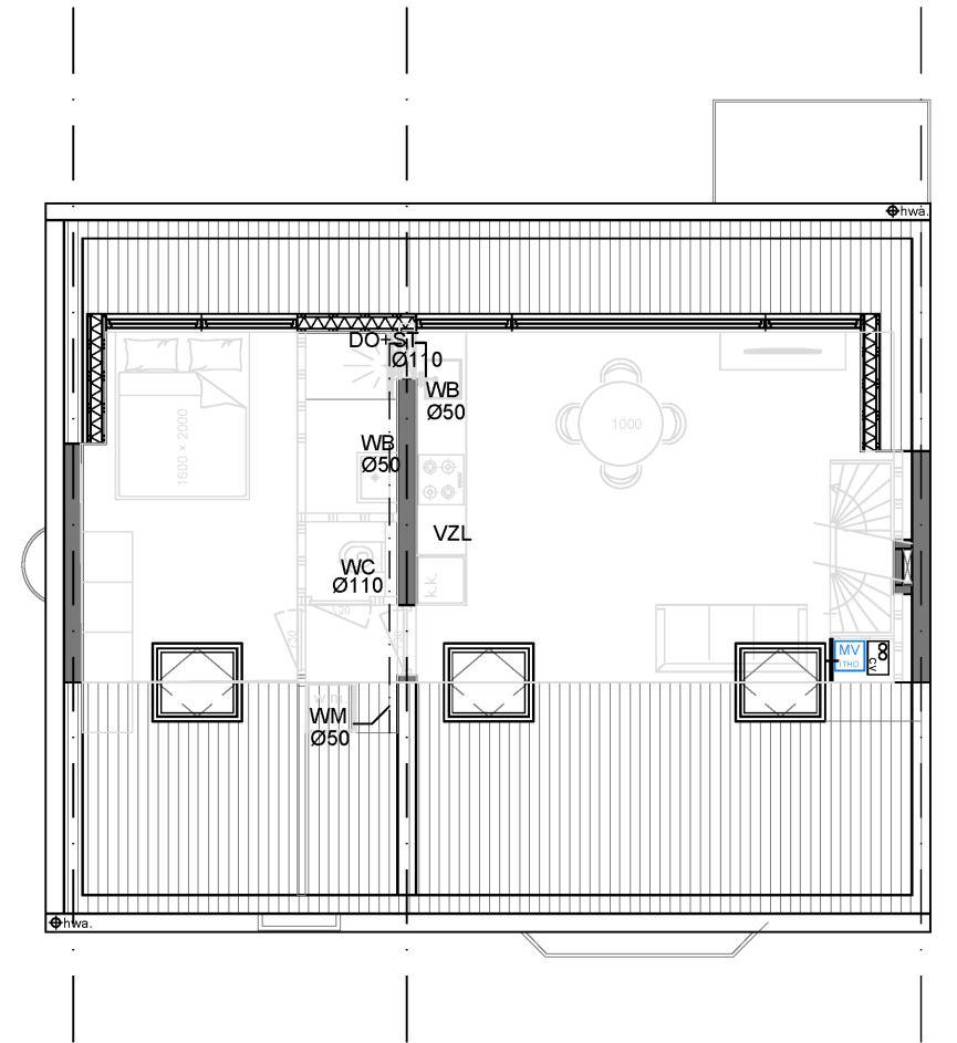
Derde verdieping
