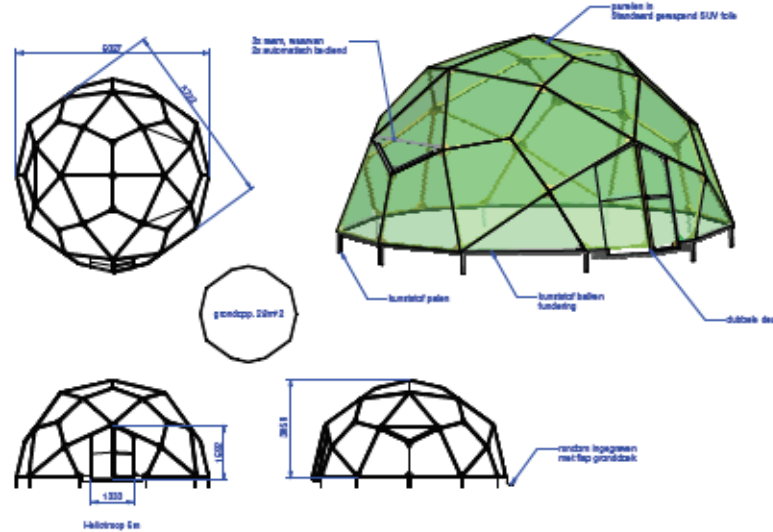
Tekening Kas
