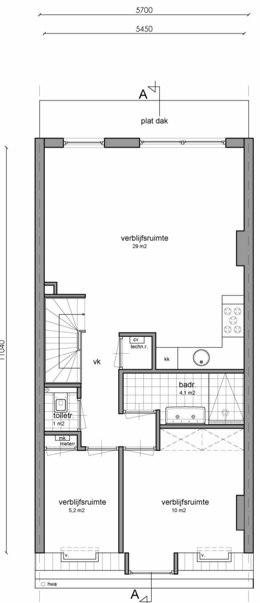
Vierde verdieping
