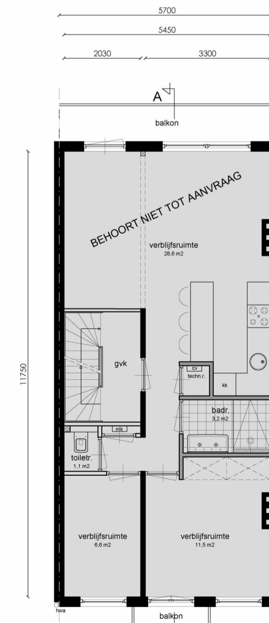
Tweede verdieping
