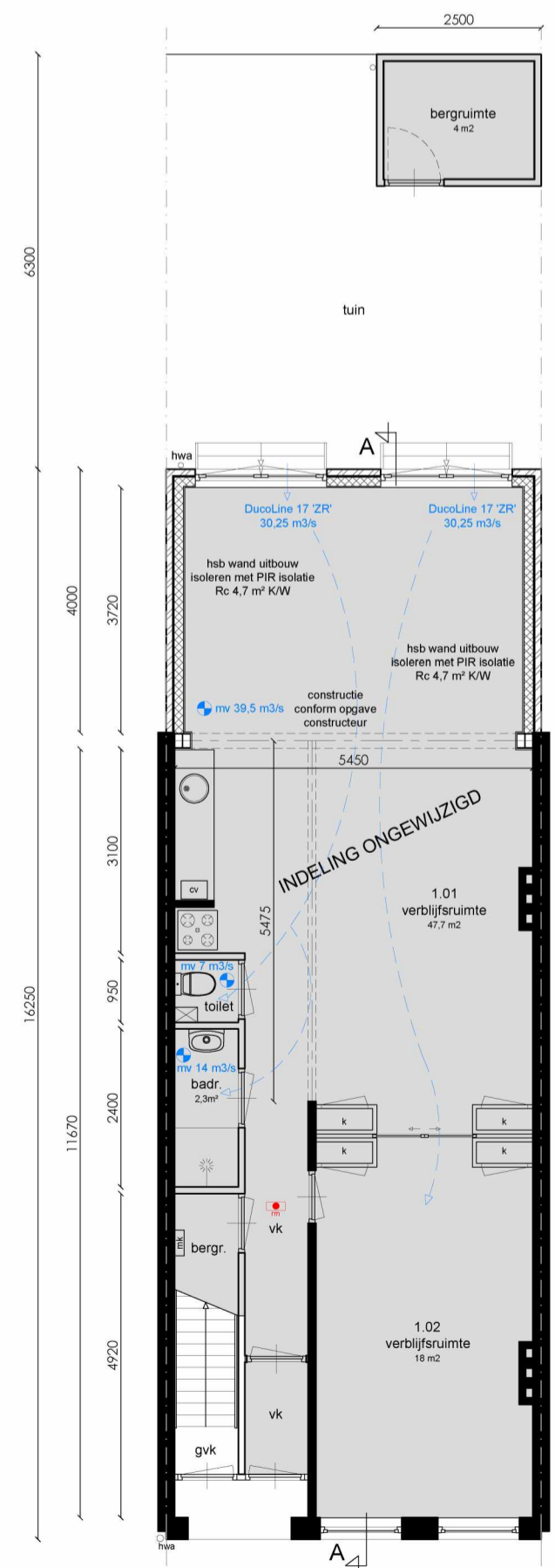
Begane grond
