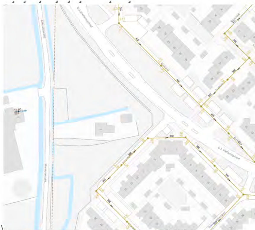
Figuur 7 Riolering ten zuidoosten van het plangebied
