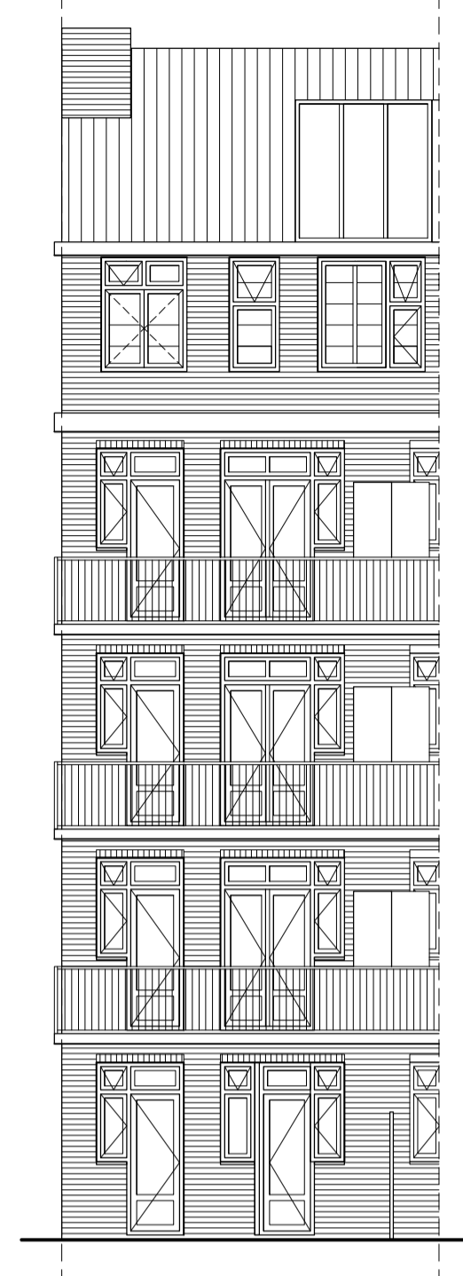
Achtergevel
