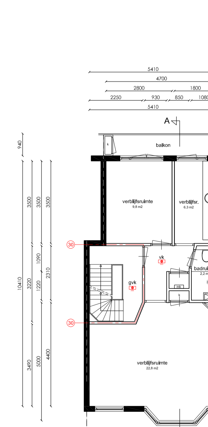
Derde verdieping
