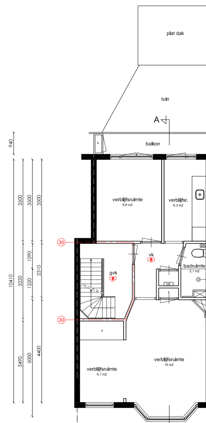
Eerste verdieping
