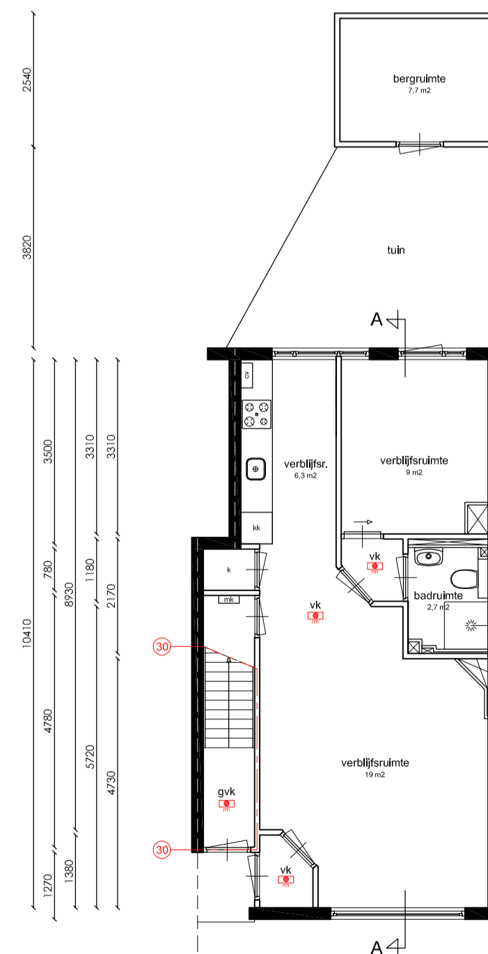
Begane grond
