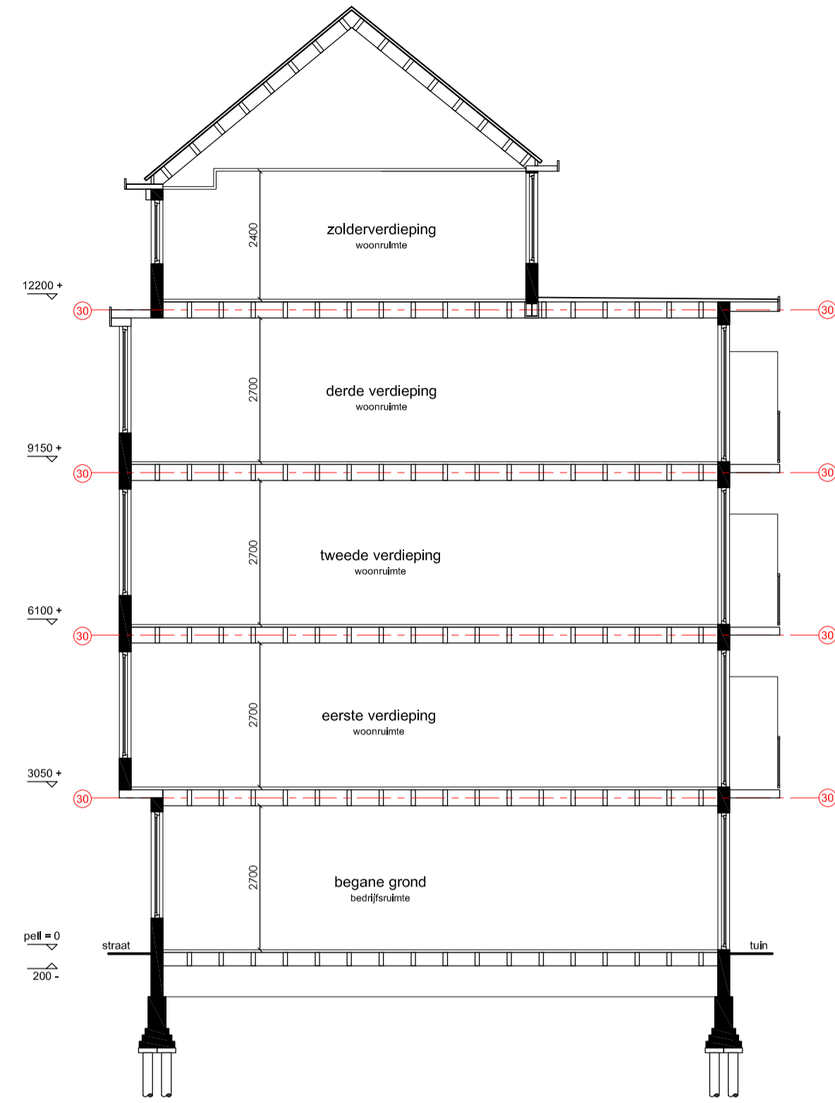
Doorsnede A-A
