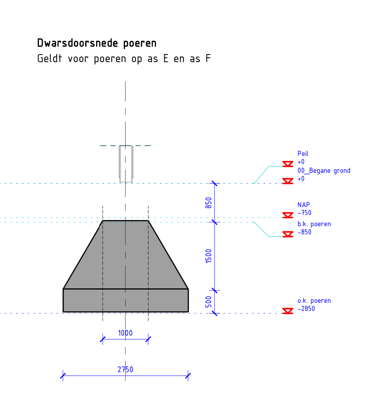
Dwarsdoorsnede poeren hal 29 1:50
