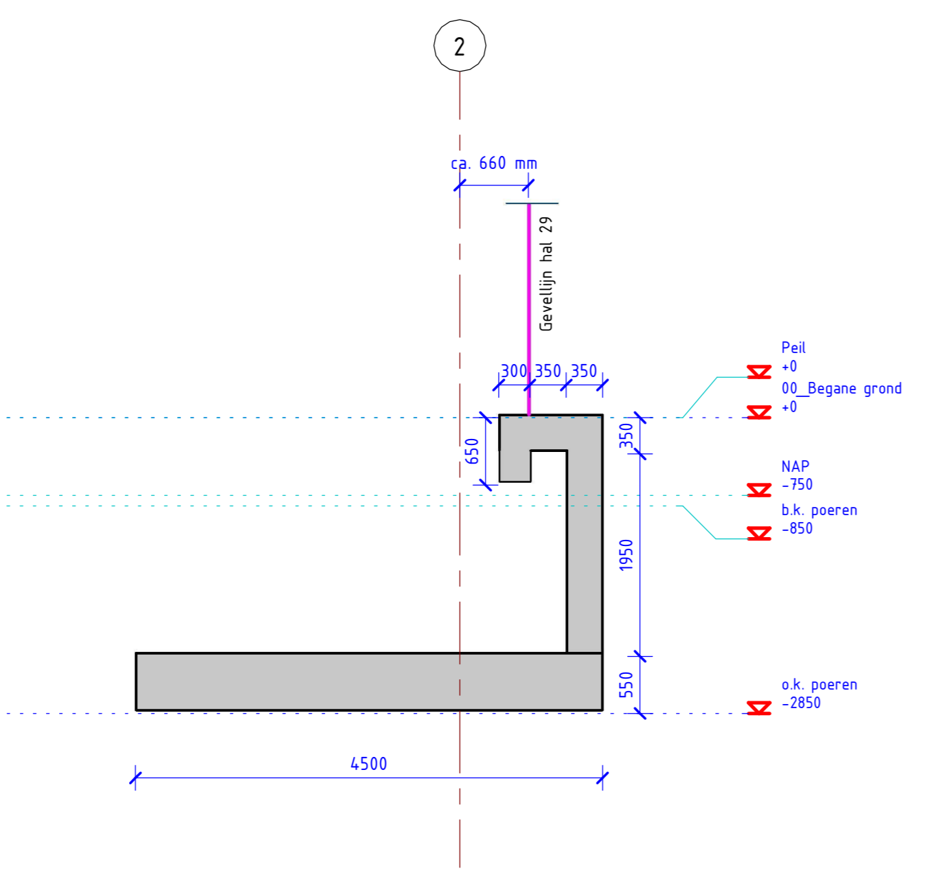
Havenconstructie 1:50
