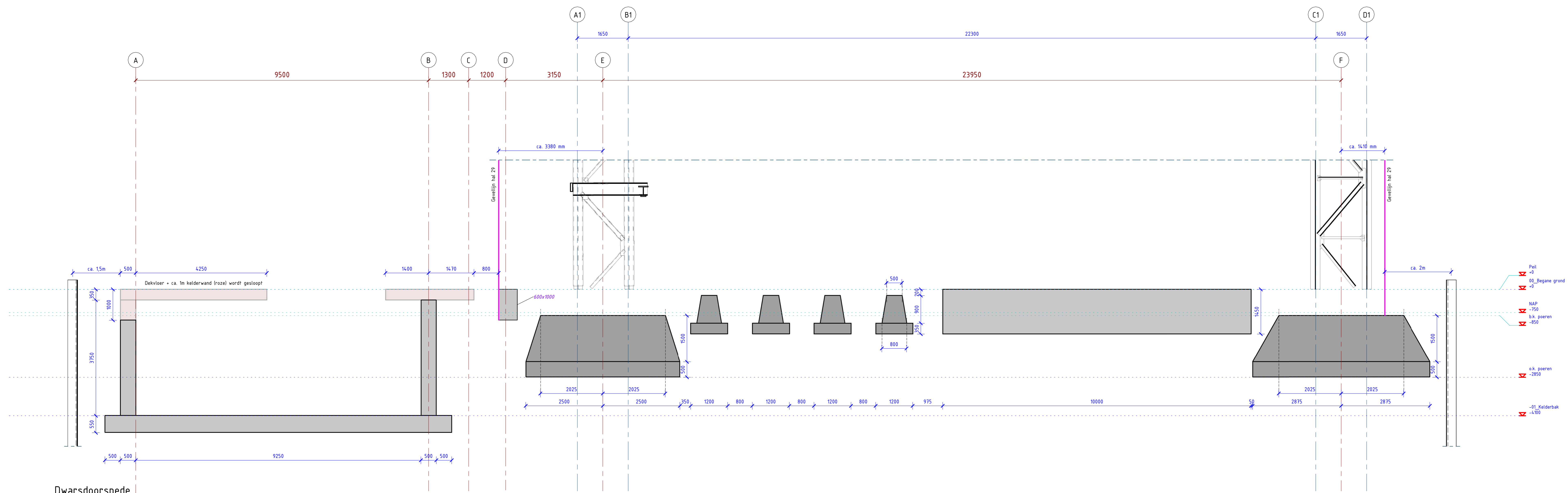
Dwarsdoorsnede 1:50
