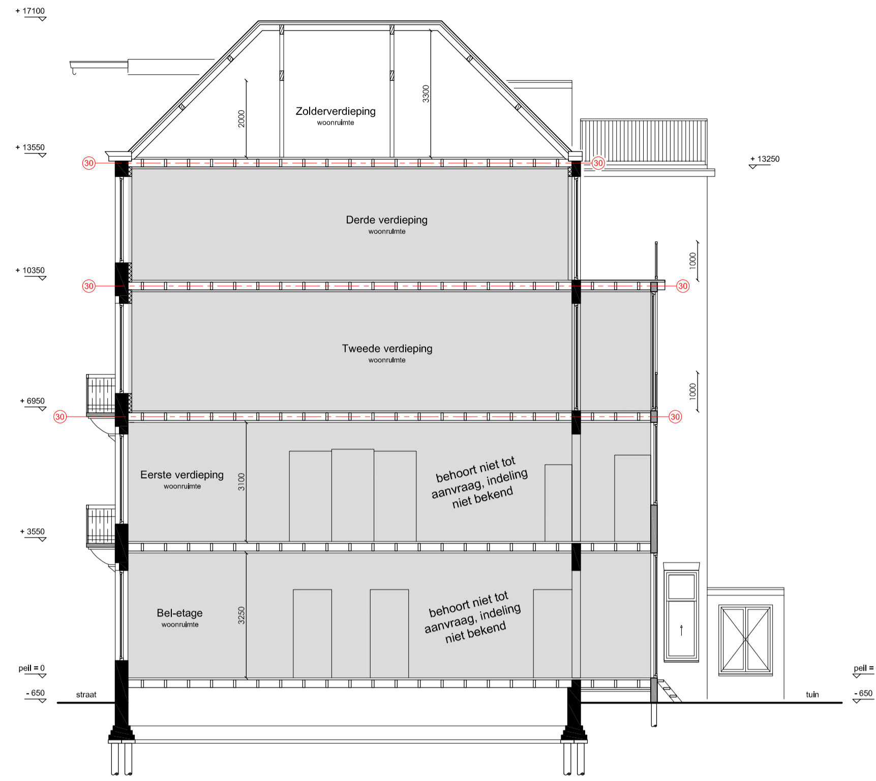
Doorsnede A-A Ongewijzigd
