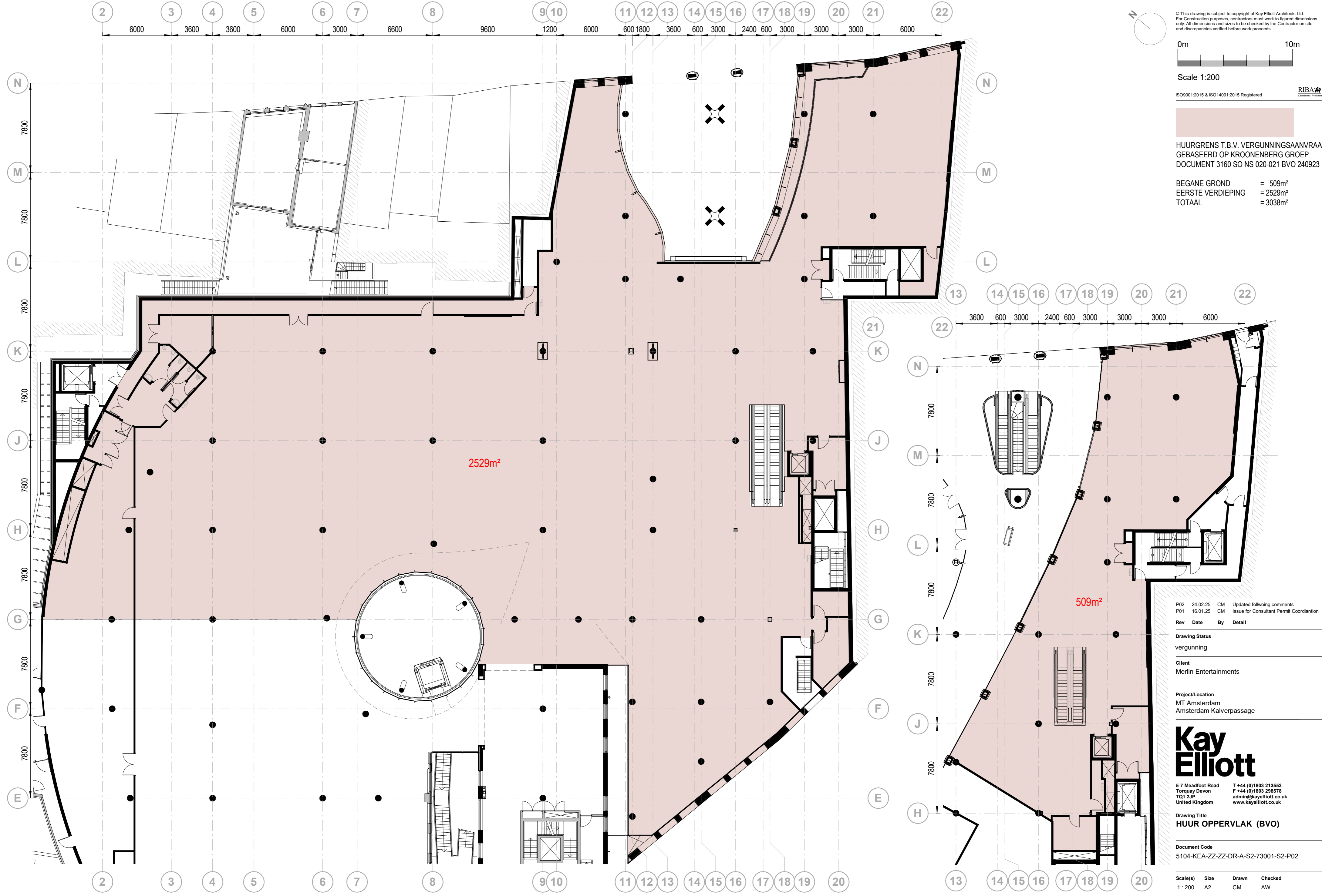
1ste Verdieping 1 : 200
